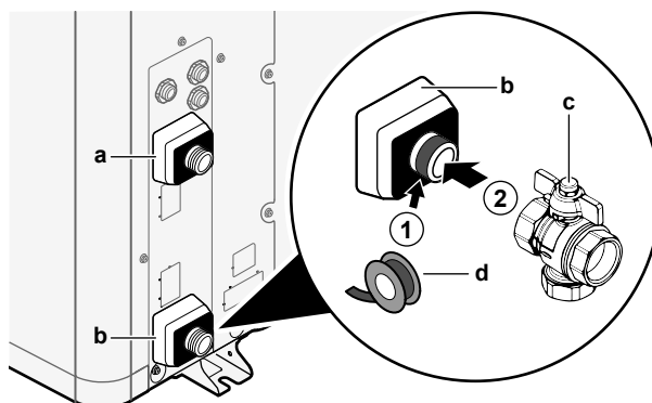
a WASSERAUSLASS (Schraubverbindung, Stecker, 1")
