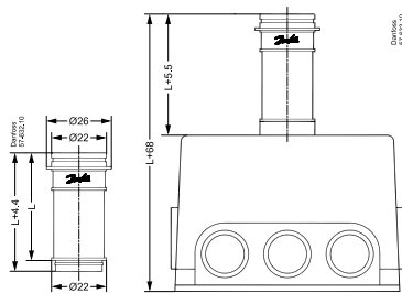
Unterteil 057H7210
