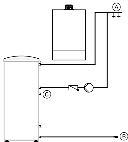
Nebengestellter Speicher-Wassererwärmer
