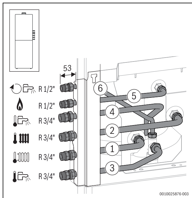
Bild 56 Zubehör CS 10 auf der rechten Seite montiert
