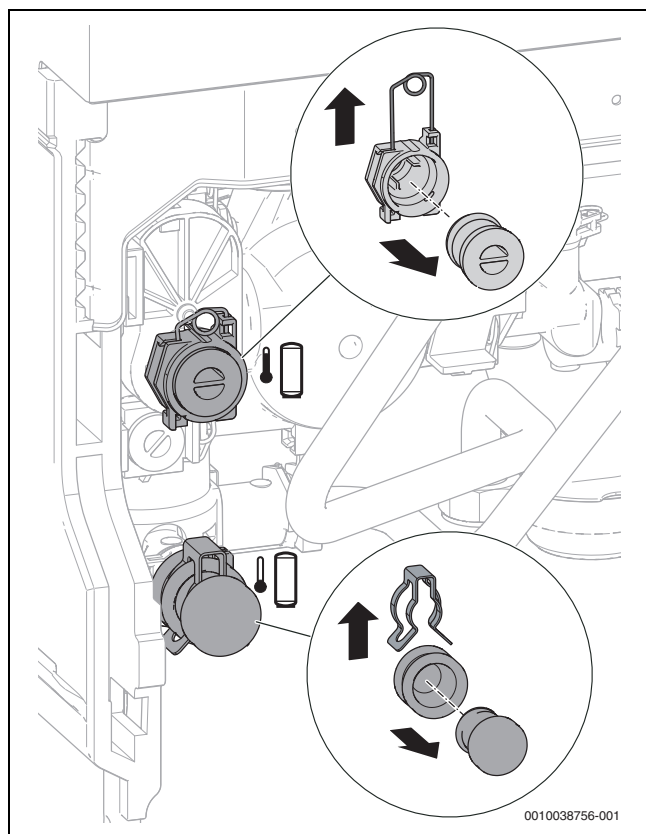
Bild 80 Stopfen abnehmen
