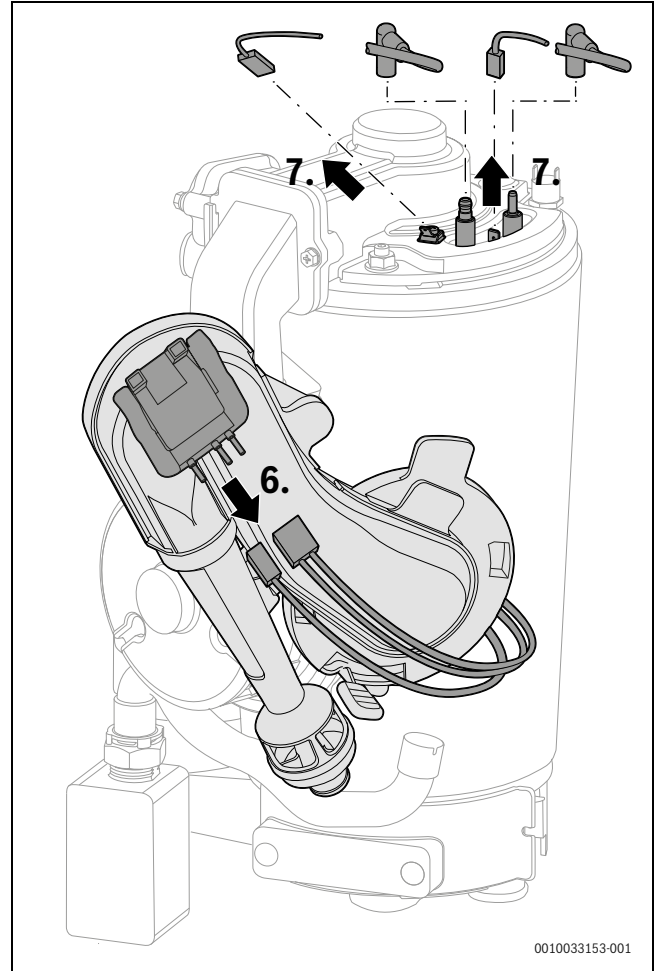
Bild 20 Kabel abziehen
