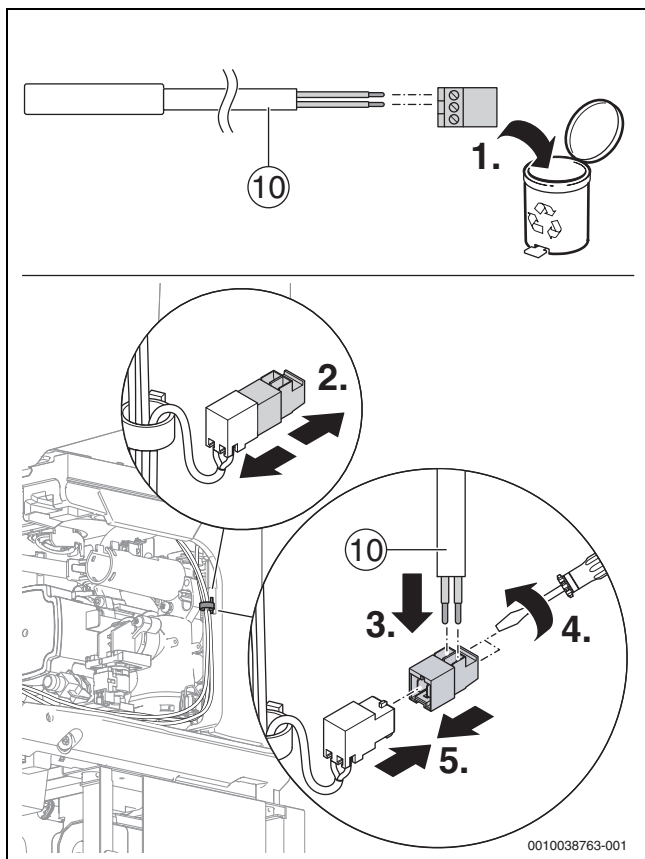
Bild 98 Pufferspeicher-Temperaturfühler anschließen
