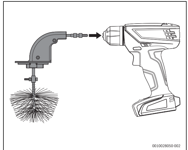
Bild 28 Bürste mit Akku-Schrauber verbinden
