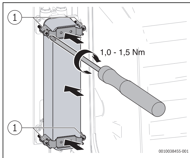
Bild 55 Plattenwärmetauscher einbauen
