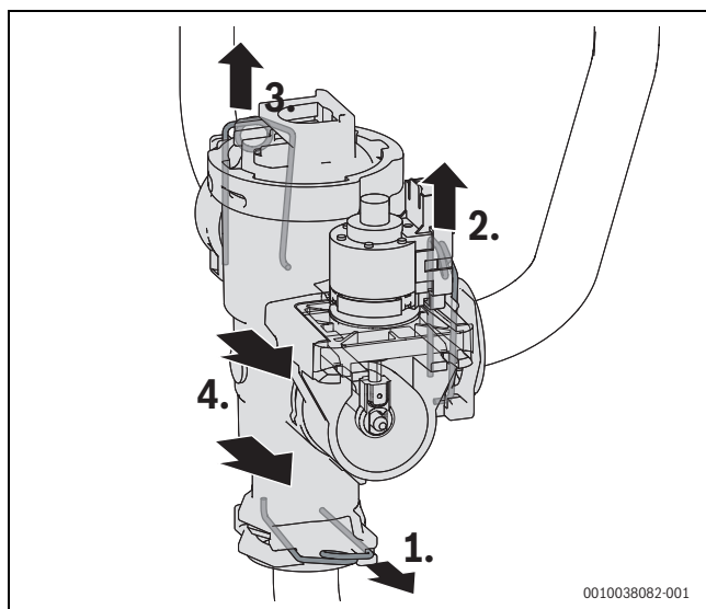
Bild 57 Federn lösen
