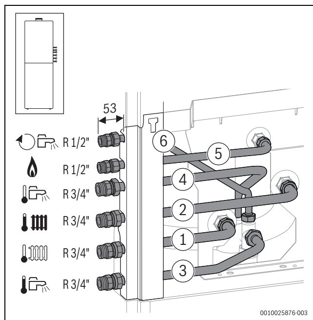
Bild 102 Zubehör CS 10 auf der rechten Seite montiert
