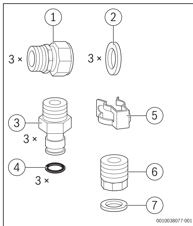
Bild 95 Lieferumfang Zubehör CS 42
