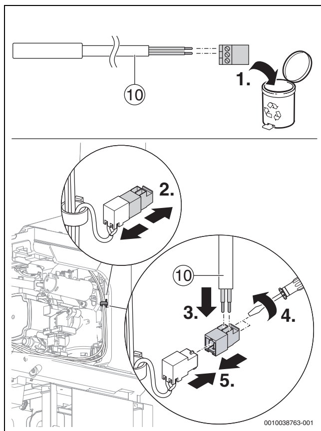
Bild 139 Pufferspeicher-Temperaturfühler anschließen
