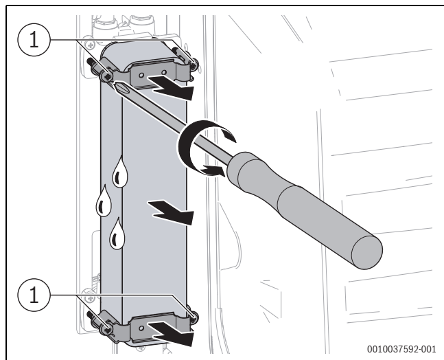
Bild 53 Plattenwärmetauscher ausbauen
