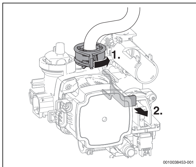
Bild 37 Heizungspumpe entriegeln
