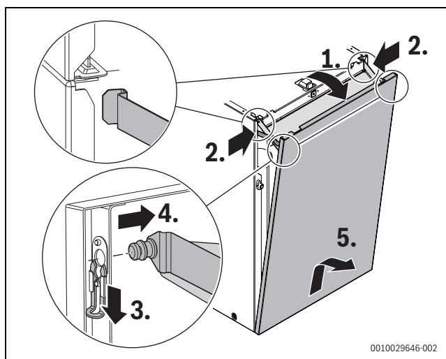
Bild 60 Vorderteil der Speicherverkleidung abnehmen und sicher abstellen
