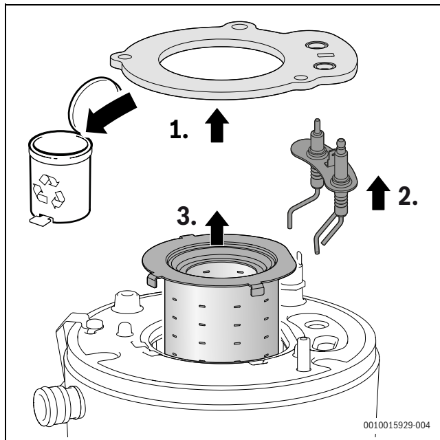
Bild 24 Brenner herausnehmen
