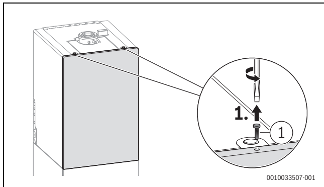
Bild 12 Sicherungsschraube lösen
