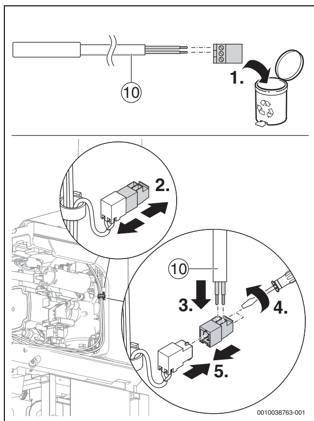
Bild 94 Pufferspeicher-Temperaturfühler anschließen
