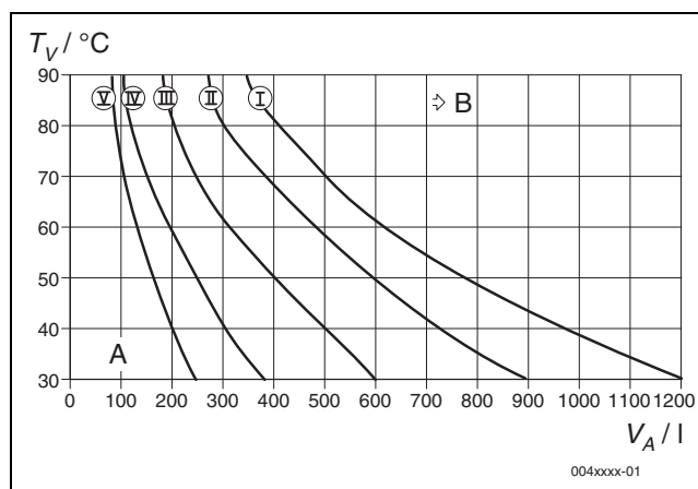
Bild 50 Größe des Ausdehnungsgefäßes für Pufferspeicher mit maximal 400 l Inhalt bestimmen
