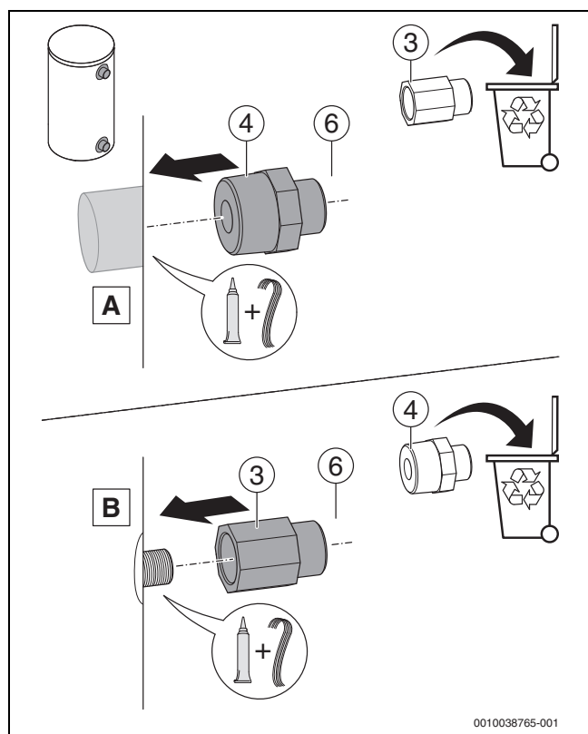
Bild 88 Adapter am oberen und unteren Anschluss des Pufferspeichers einsetzen
