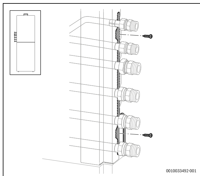
Bild 103 Abschluss der Montage auf der linken Seite
