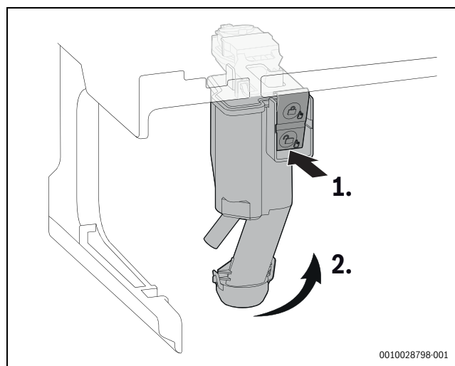
Bild 64 Kondensatsiphon herausnehmen
