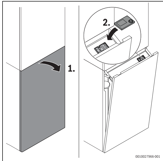
Bild 149 Bedieneinheit Logamatic RC310 einsetzen
