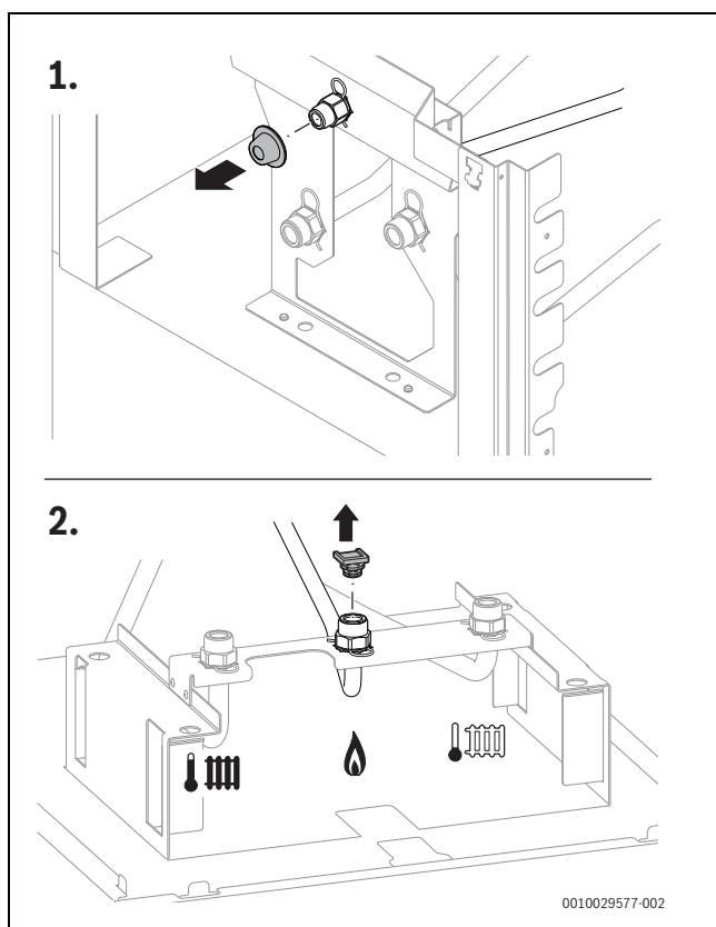
Bild 58 Schutzkappe und Stopfen am Gasrohr entfernen
