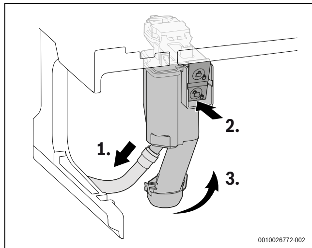
Bild 48 Kondensatsiphon ausbauen
