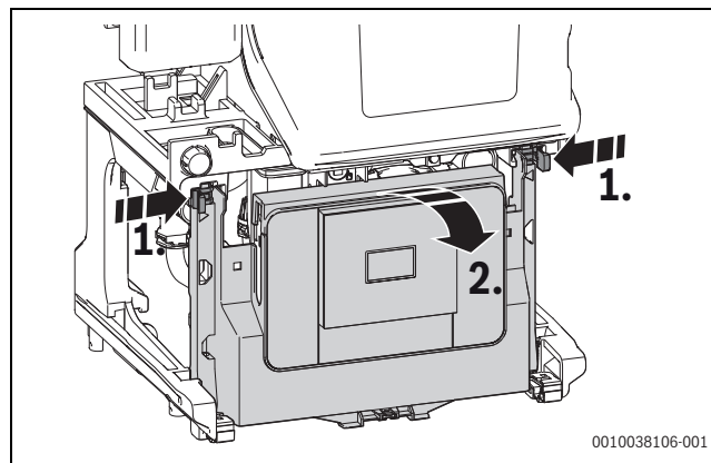
Bild 63 Steuergerät herunterklappen
