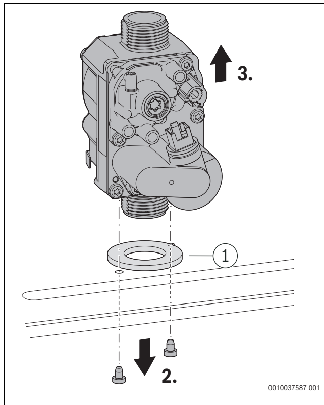
Bild 42 Gasarmatur ausbauen
