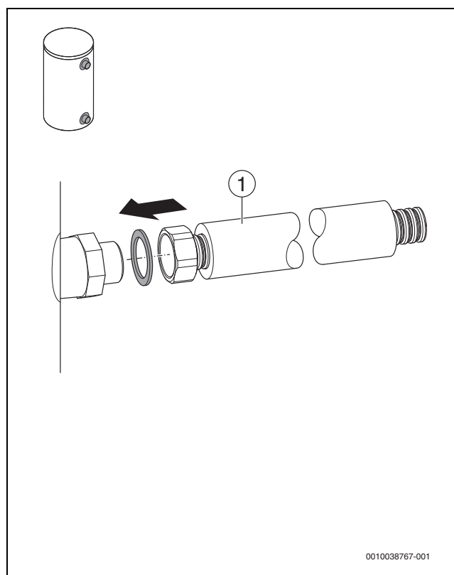
Bild 89 Verbindungsleitungen am Pufferspeicher anschließen
