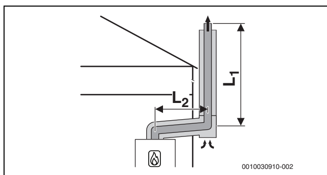
Bild 34 Konzentrische Luft-Abgas-Führung nach C 53x an der Außenwand
