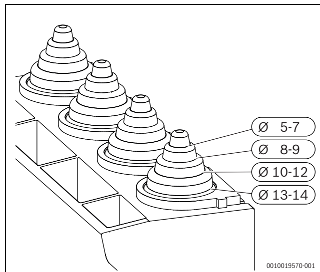
Bild 135 Zugentlastung an Kabeldurchmesser anpassen
