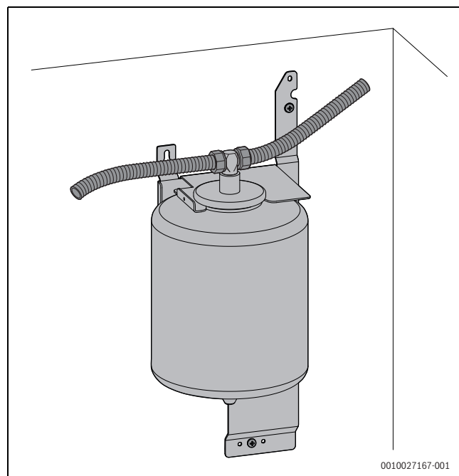
Bild 111 Zubehör EVW 8 an der Wand montiert
