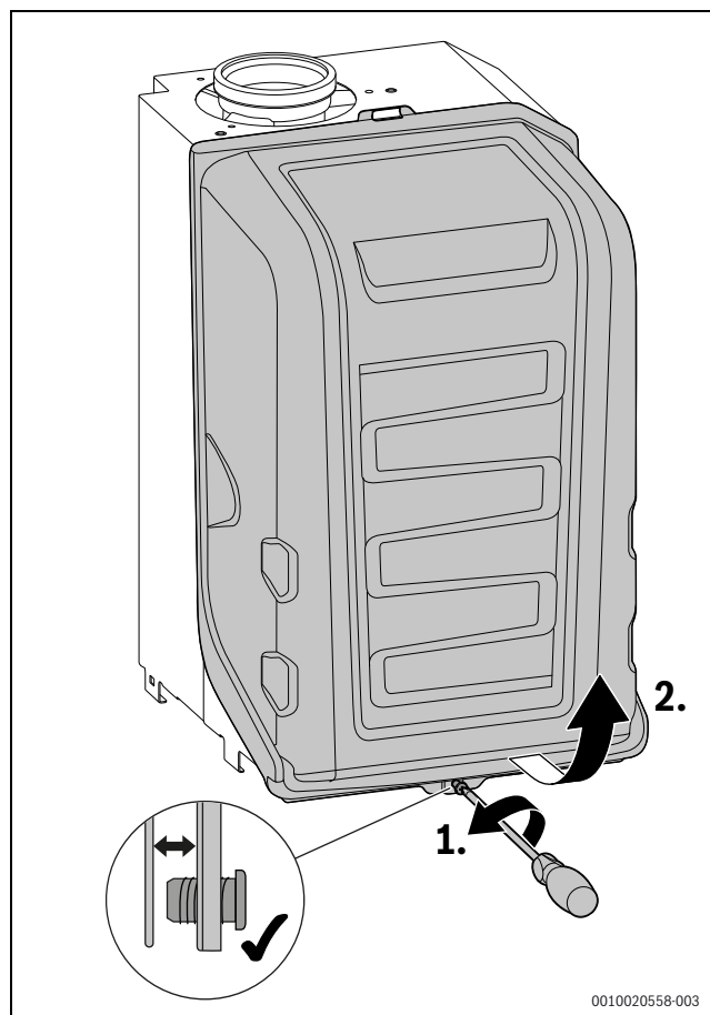
Bild 3 Brennerhaube abnehmen
