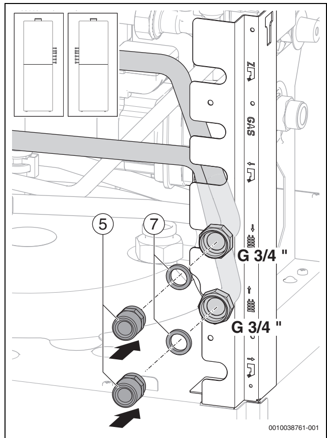
Bild 84 Doppelnippel einsetzen
