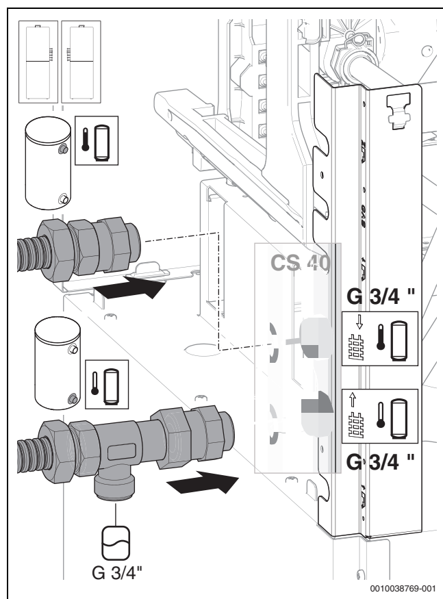
Bild 51 Ausdehnungsgefäß anschließen
