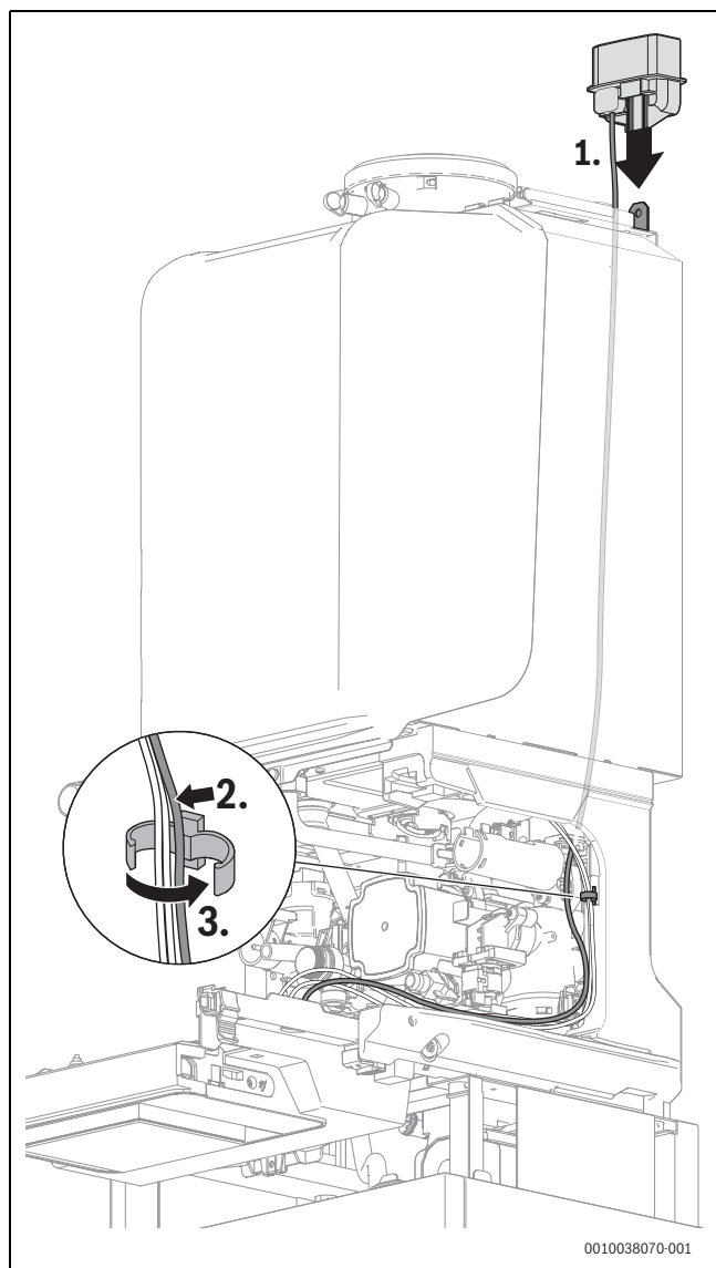
Bild 70 Funkmodul-Halter in den Steckplatz einsetzen und Kabel im Kabelhalter befestigen
