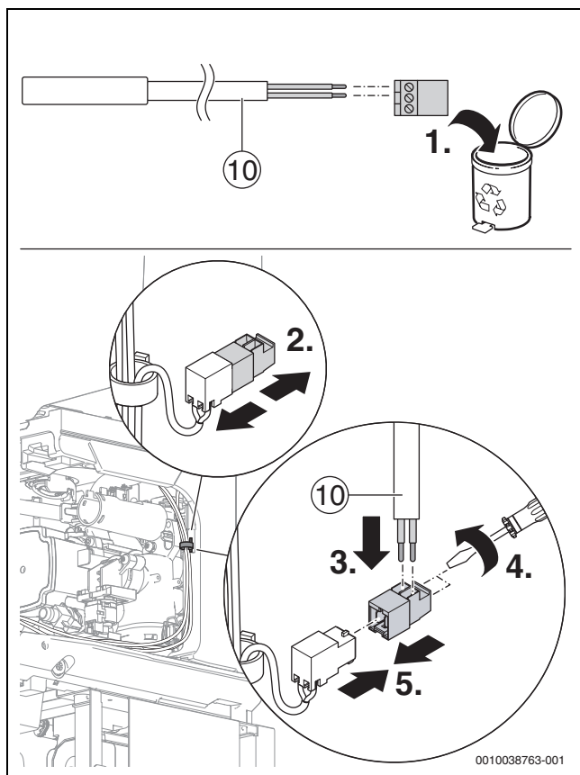
Bild 86 Pufferspeicher-Temperaturfühler anschließen
