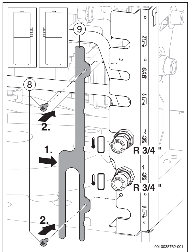
Bild 85 Halter einsetzen
