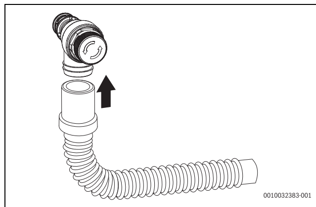
Bild 73 Schlauch am Sicherheitsventil (Heizung) montieren
