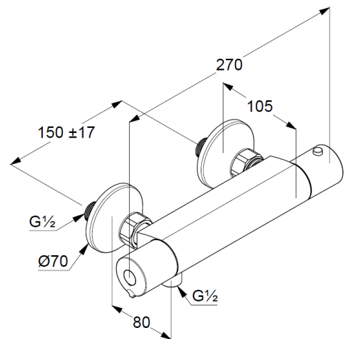
Maßzeichnung
