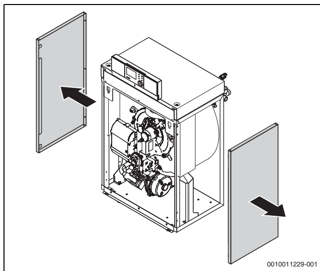
Bild 85 Seitenwände abnehmen
