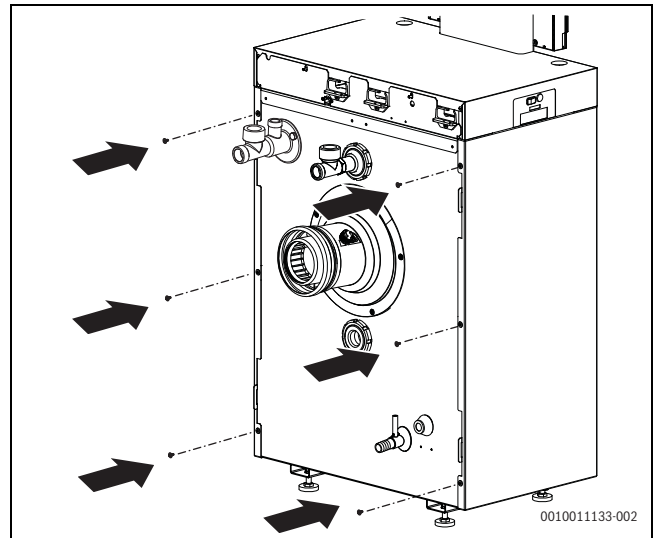
Bild 88 Seitenwände befestigen
