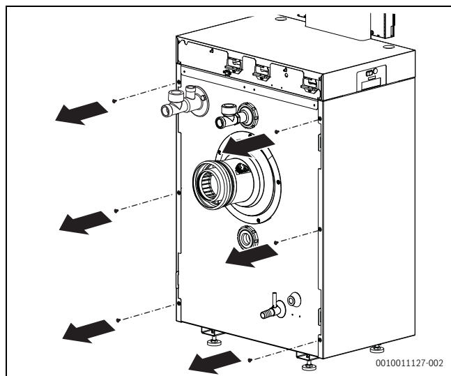
Bild 82 Befestigungsschrauben lösen
