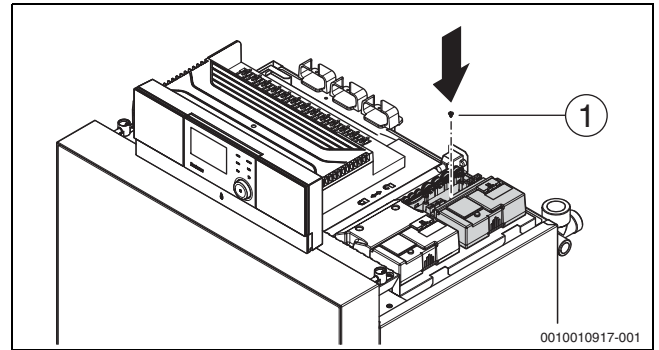
Bild 34 Funktionsmodul verschrauben
