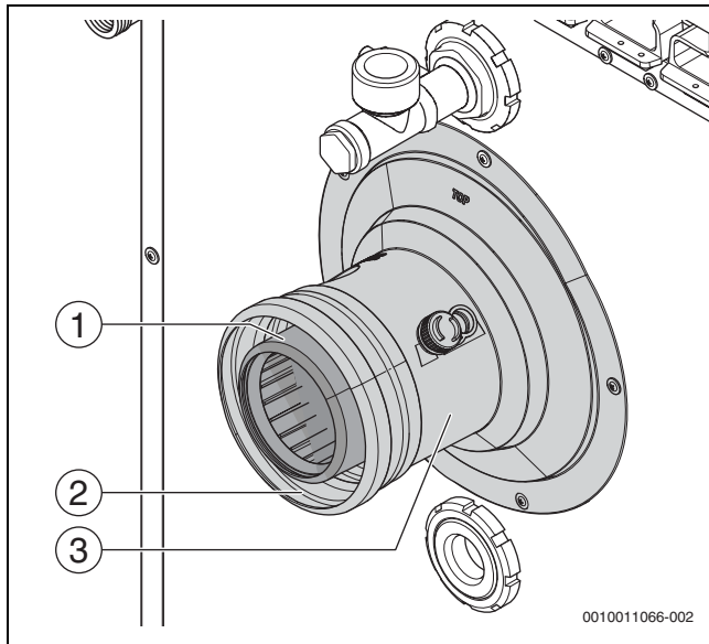
Bild 11 Abgasanschluss montieren
