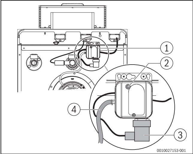
Bild 91 Abgas-Druckwächter
