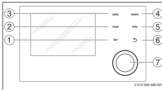
Bild 40 Bedienelemente
