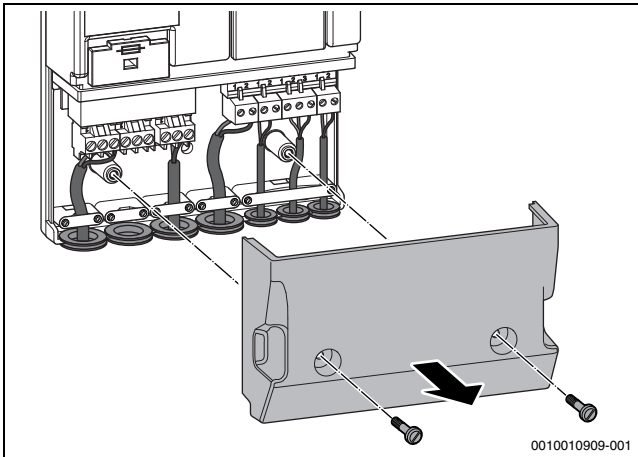
Bild 31 Funktionsmodul öffnen
