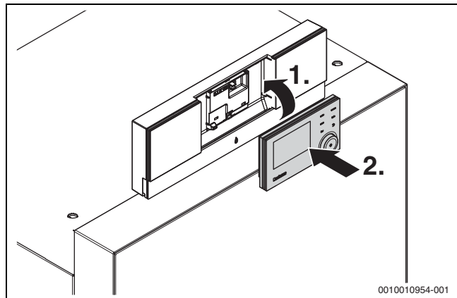
Bild 38 Bedieneinheit montieren
