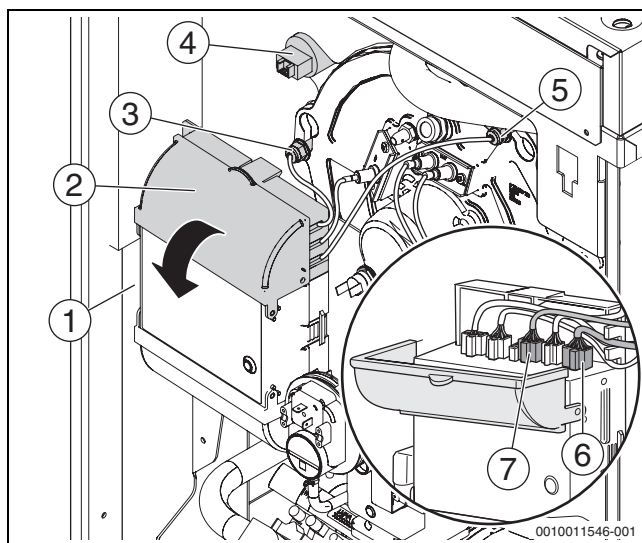
Bild 70 Steckverbinder lösen
