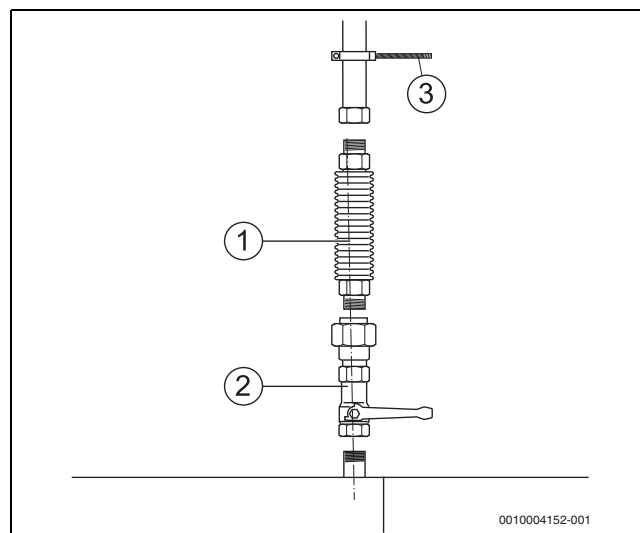
Bild 18 Gasanschluss herstellen
