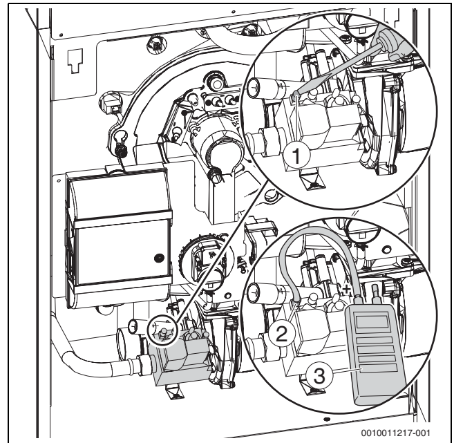
Bild 67 Gas-Anschlussdruck messen
