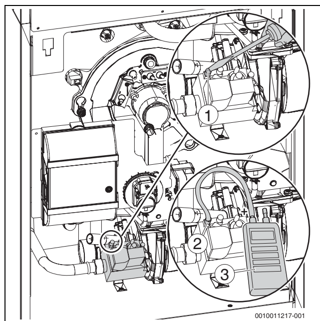
Bild 52 Gas-Anschlussdruck messen
