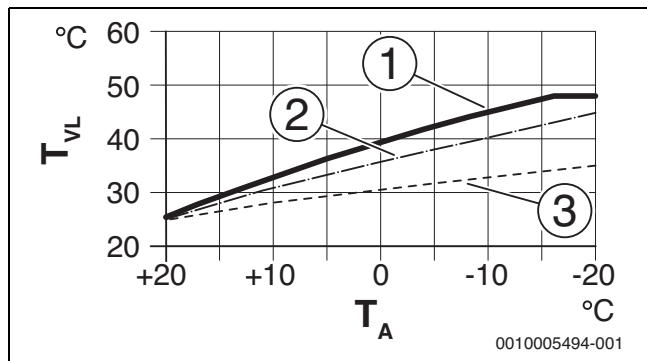
Bild 60 Einstellung der Heizkurve für Fußbodenheizung Steigung über Auslegungstemperatur T_{AL} und minimale Außentemperatur T_{A,min}
