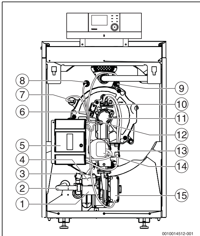
Bild 103 Vorderansicht
