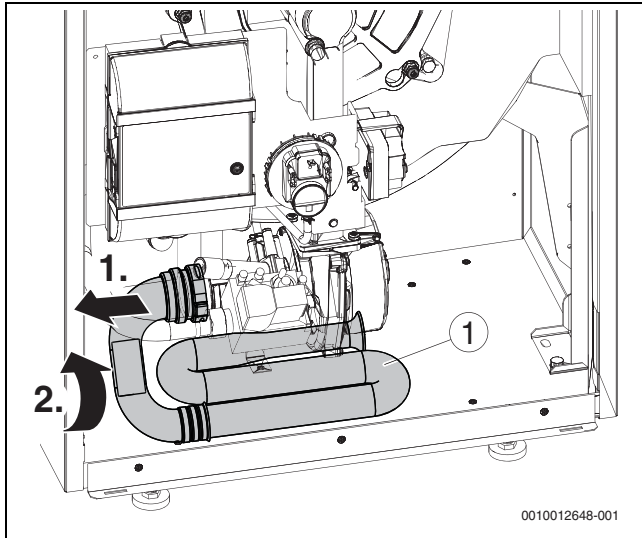
Bild 71 Ausbau Verbrennungsluft-Ansaugrohr
