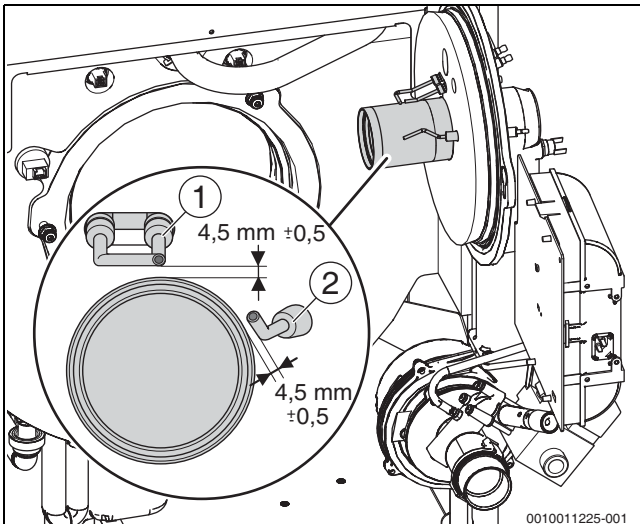
Bild 80 Abstände Elektroden
