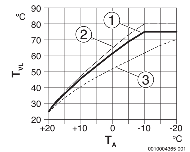
Bild 62 Einstellung der Heizkurve für Heizkörper Steigung über Auslegungstemperatur T_{AL} und minimale Außentemperatur T_{A,min}
