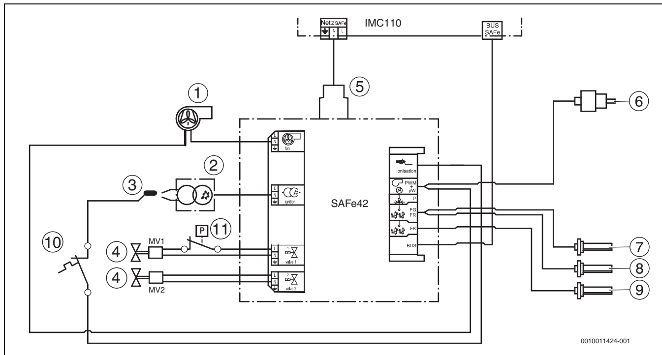
Bild 99 Anschlussplan Feuerungsautomat SAFe 42 (15...30 kW; auch 40 und 50 kW bei manchen Modellen)
