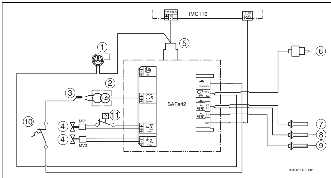
Bild 100 Anschlussplan Feuerungsautomat SAFe 42 (40 kW und 50 kW; nicht bei allen Modellen)
