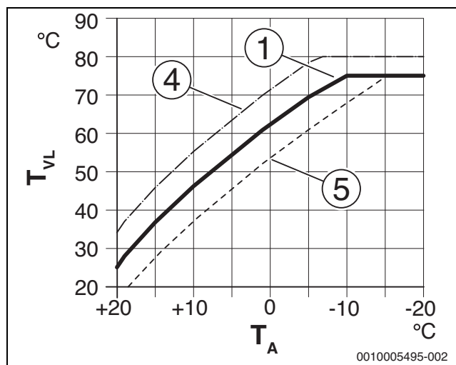
Bild 63 Einstellung der Heizkurve für Heizkörper Parallelverschiebung über Raumtemperatur-Offset oder gewünschte Raumtemperatur
