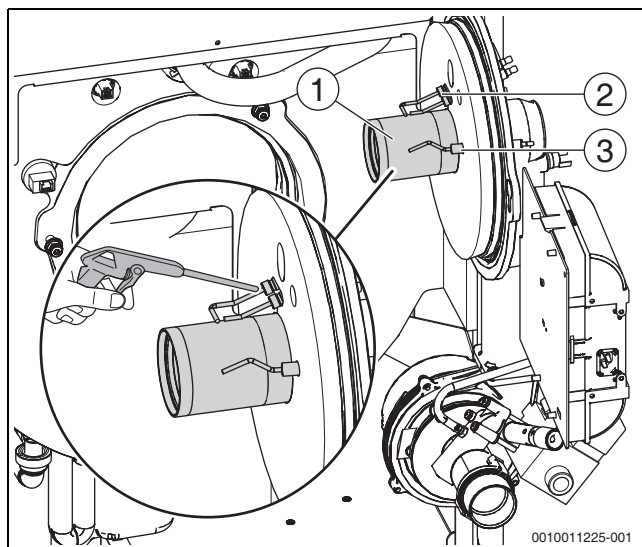
Bild 78 Brennerrohr mit Druckluft ausblasen
