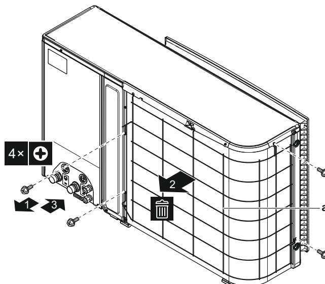
a Ansaugluftgitter
