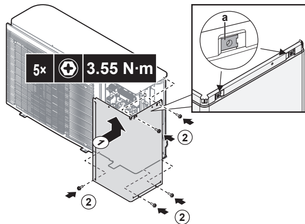
a Blechmutter
