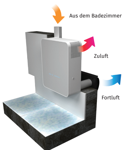
Funktionsweise mit zusätzlichem Anschlussstutzen zur Entlüftung von Badezimmern
