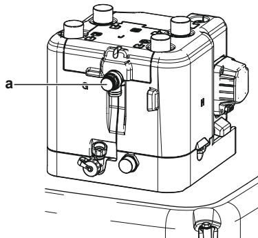
a Druckentlastungsventil
