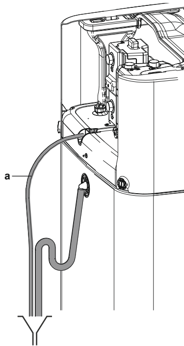
a Ablaufwannenschlauch
