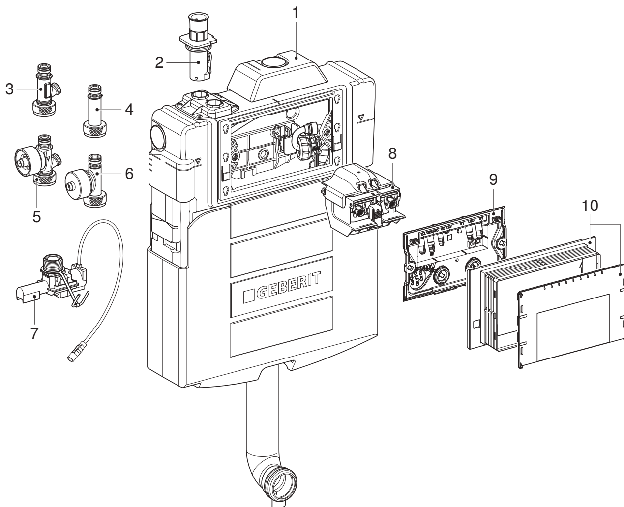
Slika 1: Higijenski splakovanji Geberit HS30 in HS50 v podometnem splakovalniku
