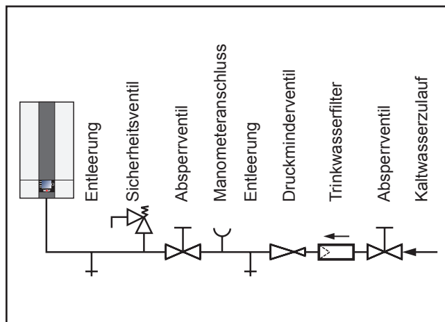
Bild: Kaltwasseranschluss nach DIN 1988
