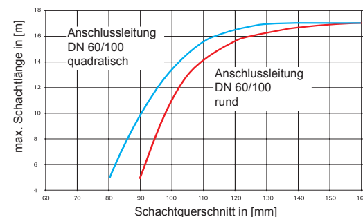
Abgasrohr DN 60
