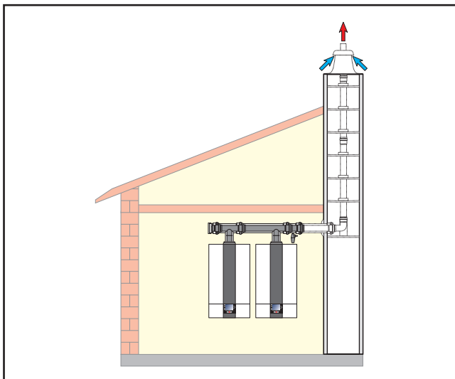
Bild: Kaskade
