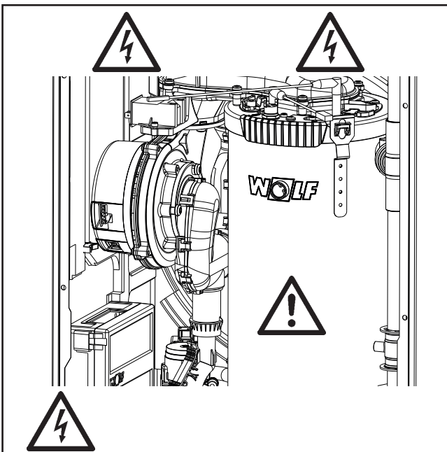
Bild: Zündtrafo, Hochspannungs-Zündeletrode, Brennkammer Gefahr durch elektrische Spannung, Gefahr von Verbrennung durch heiße Bauteile
