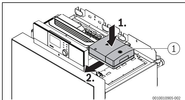
Bild 39 Funktionsmodule einstecken
