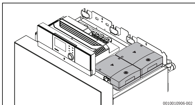
Bild 40 Standard-Funktionsmodule montiert
