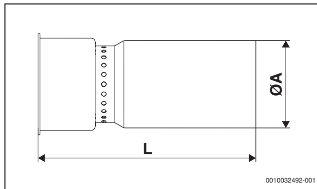
Bild 96 Brennerrohre
