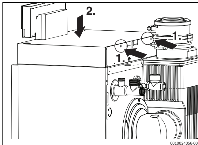
Bild 38 Kesselhaube montieren
