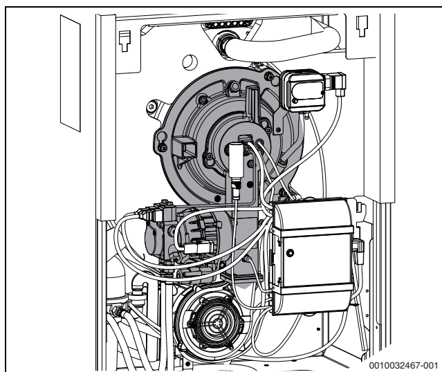
Bild 56 Heiße Bauteile am Brenner/Wärmetauscher
