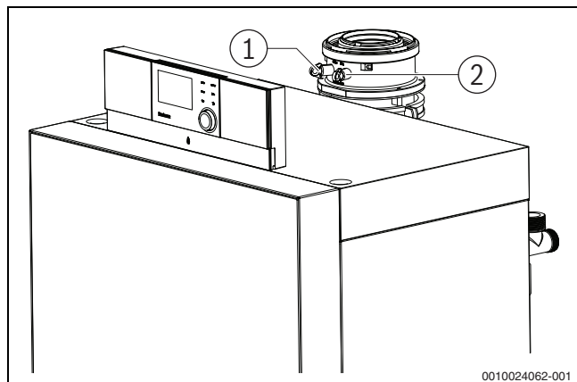
Bild 55 Messwerte aufnehmen
