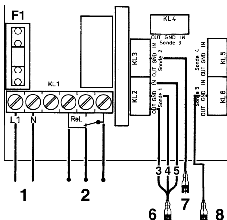
Figura 6: Allacciamento elettrico OM 5
