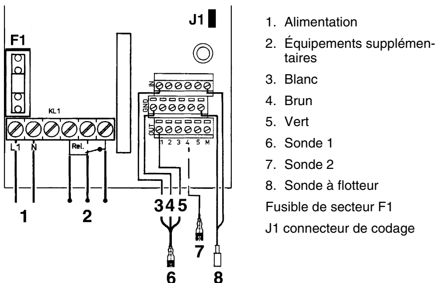
Figure 7: Branchement électrique OM 5+1
