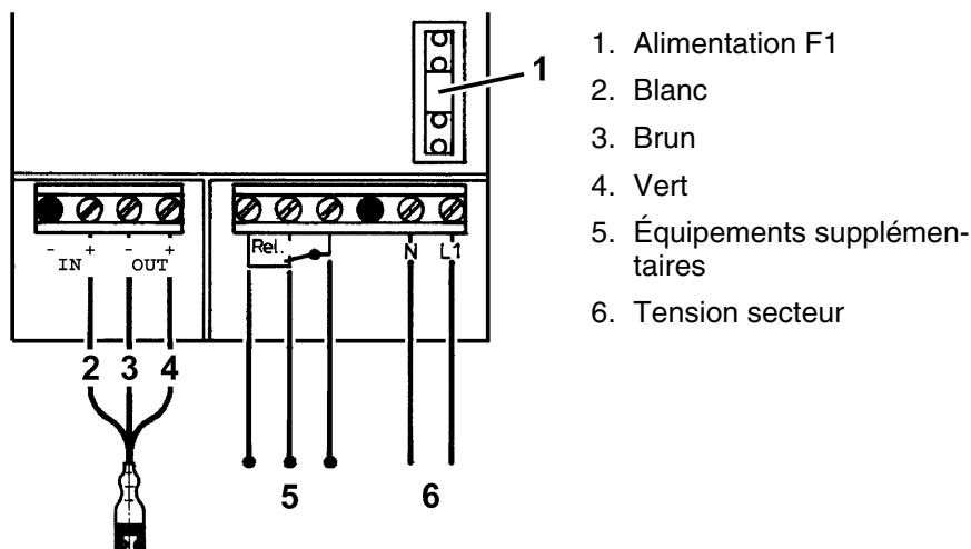
Figure 8: Branchement électrique OM 1
