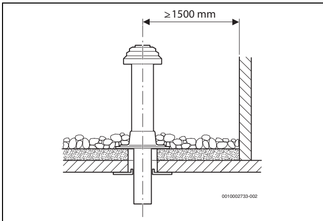
Bild 12 Abstandsmaß bei Flachdach
