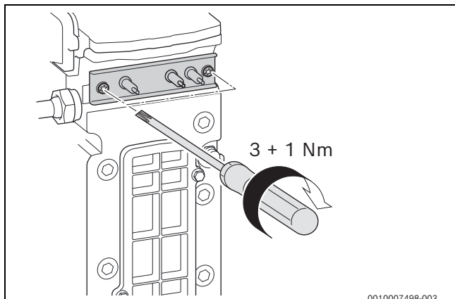
Bild 79 Elektroden-Set montieren
