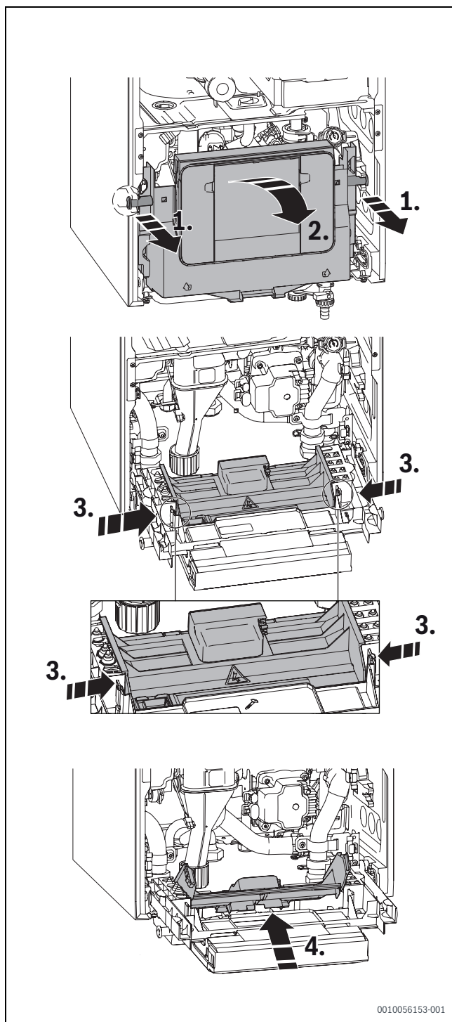
Bild 63 Steuergerät öffnen
