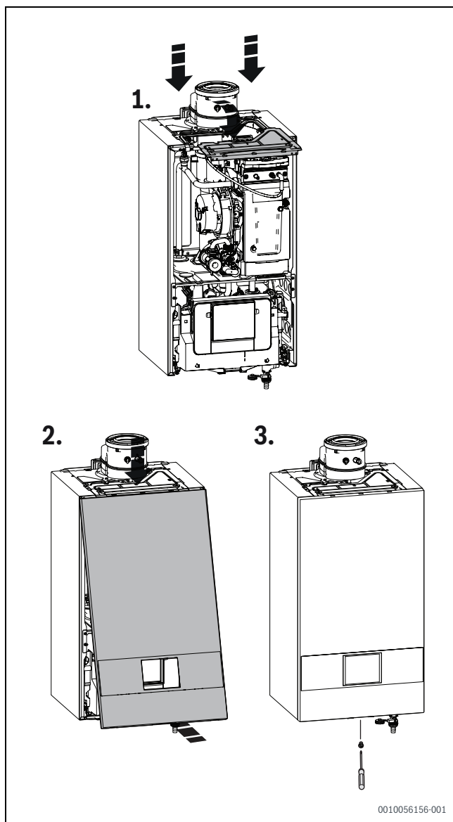
Bild 68 Verkleidung montieren
