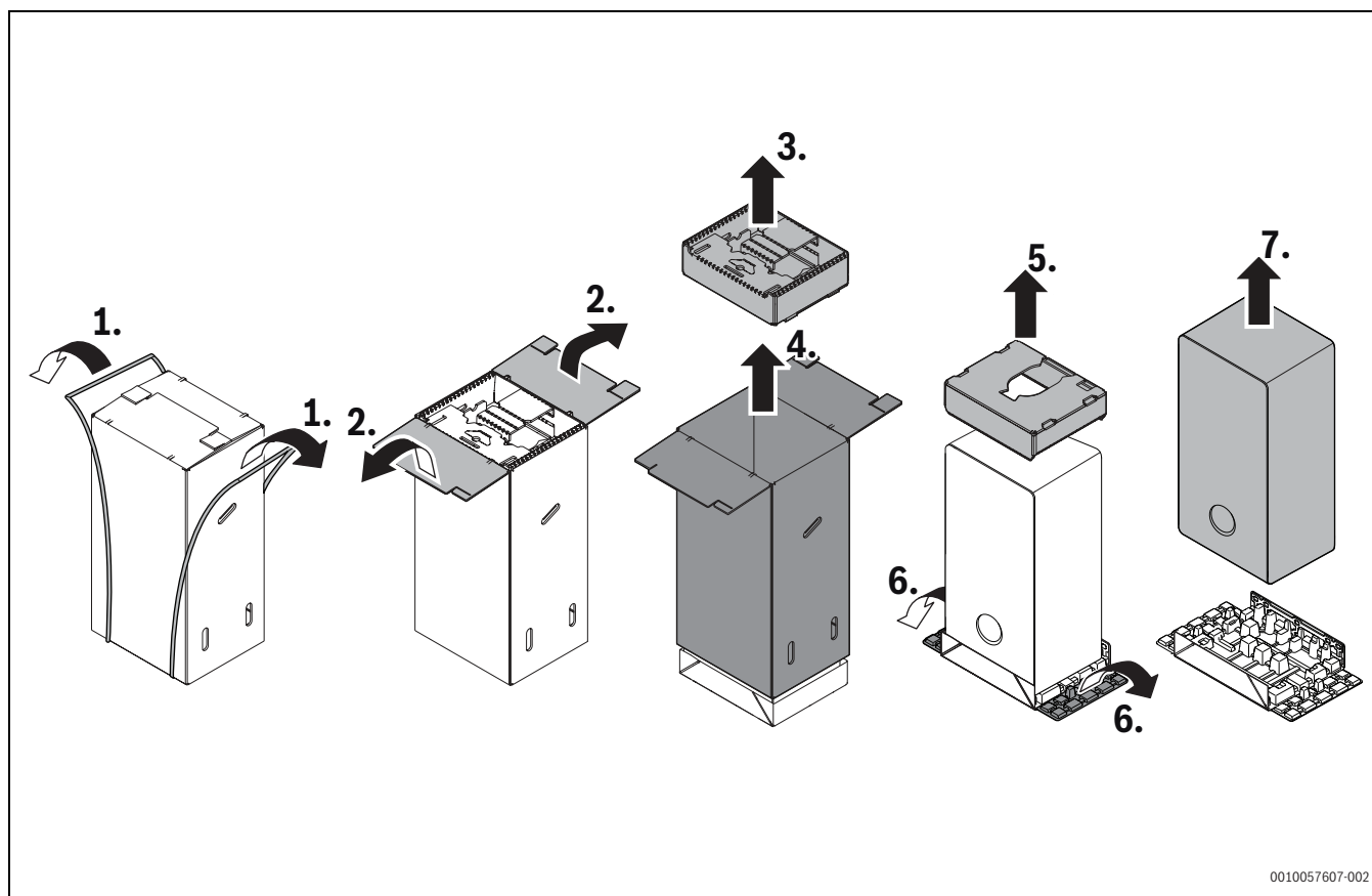
Bild 38 Auspackanweisung
