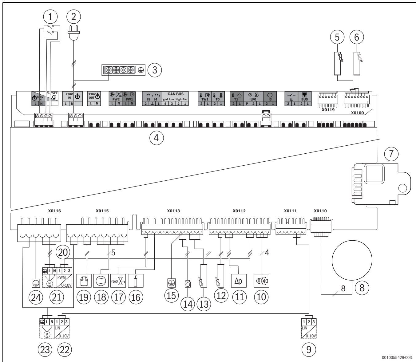
Bild 106 Elektrische Verdrahtung
