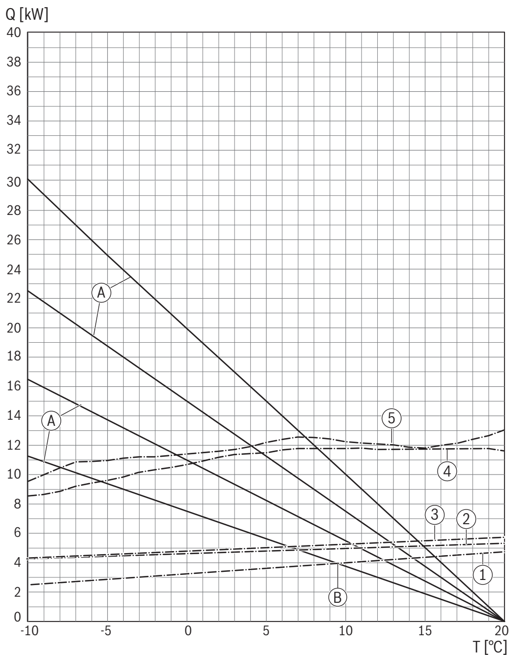
Bild 73 Diagramm für Tabelle 95 zur Bestimmung der Bivalenztemperaturen bei einer Vorlauftemperatur von 65 °C
