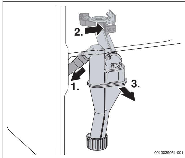
Bild 95 Kondensatsiphon ausbauen
