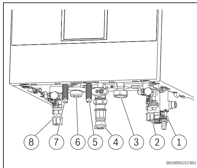
Bild 61 Gas- und wasserseitige Anschlüsse (Zubehör)
