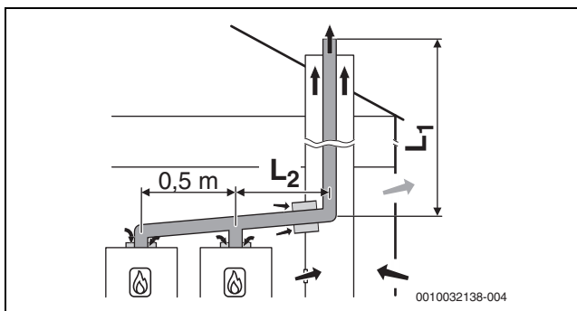
Bild 34 Kaskade mit 2 Geräten:
