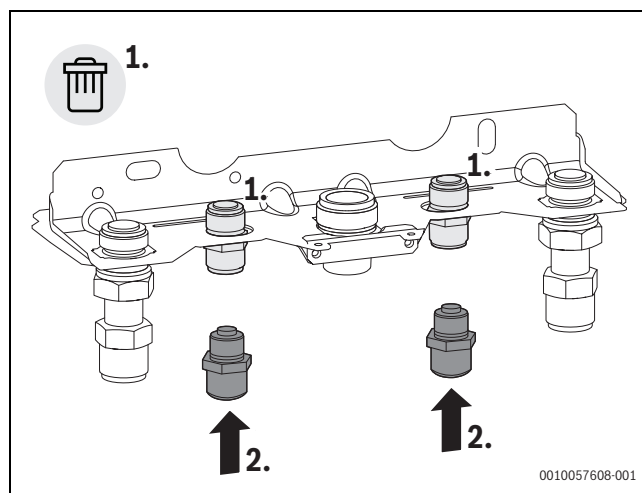
Bild 51 Anschlussadapter (7738112656) ersetzen
