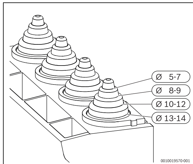
Bild 64 Zugentlastung an Kabeldurchmesser anpassen
