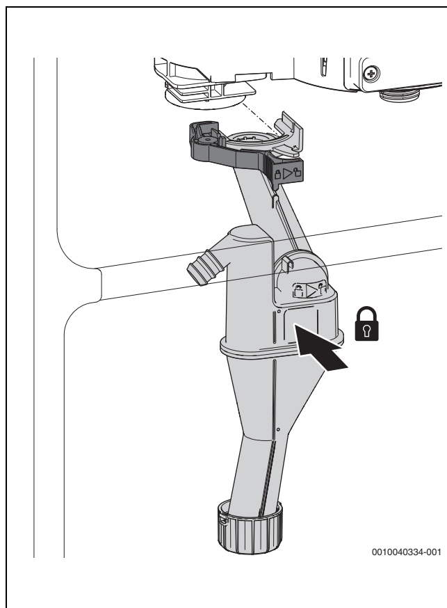
Bild 99 Kondensatsiphon einsetzen
