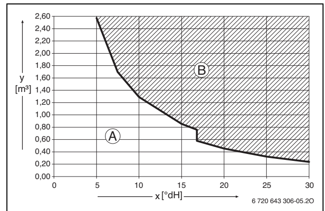
Bild 37 Anforderungen an Füll- und Ergänzungswasser Geräte < 50 kW
