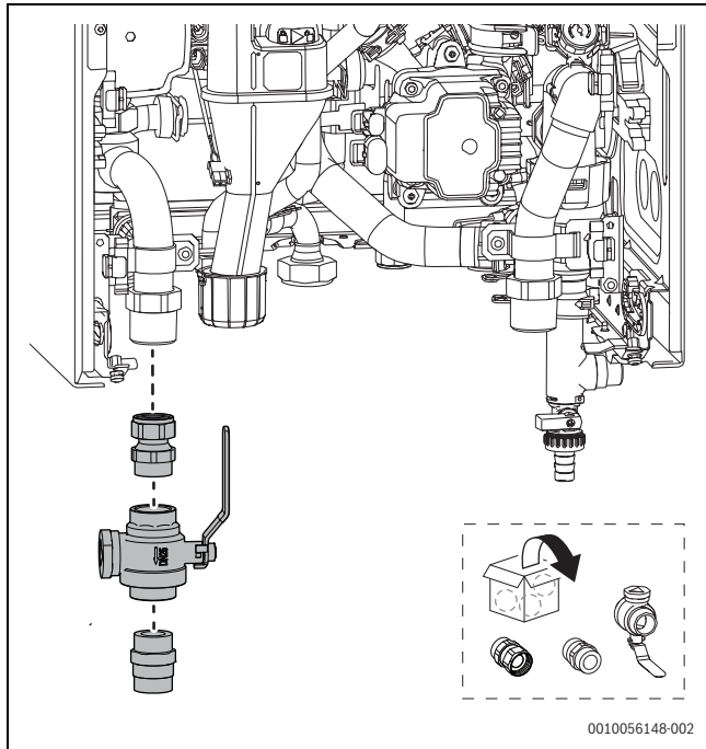
Bild 46 Partikelfilter installieren
