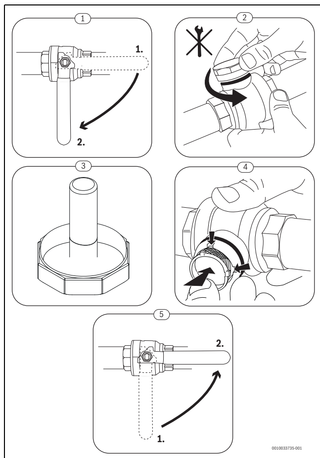
Bild 100 Siebreinigung
