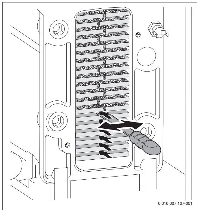
Bild 91 Reinigungsmesser
