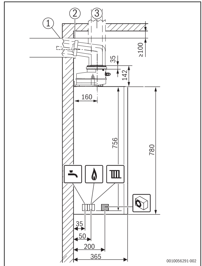
Bild 2 Seitenansicht (mm)
