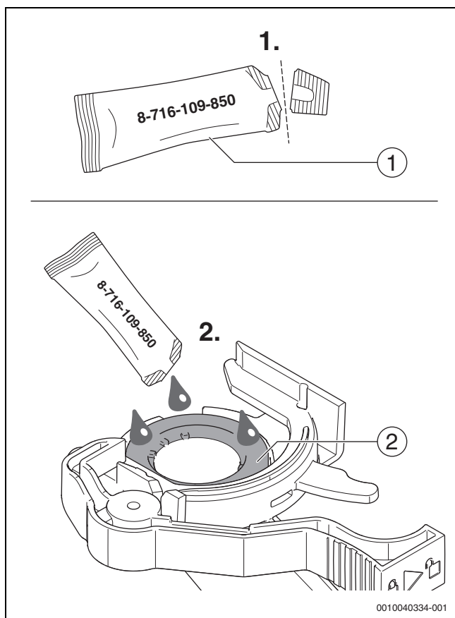
Bild 98 Dichtung fetten
