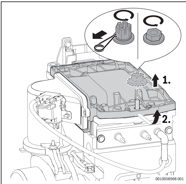
Bild 84 Brennerdeckel ausbauen
