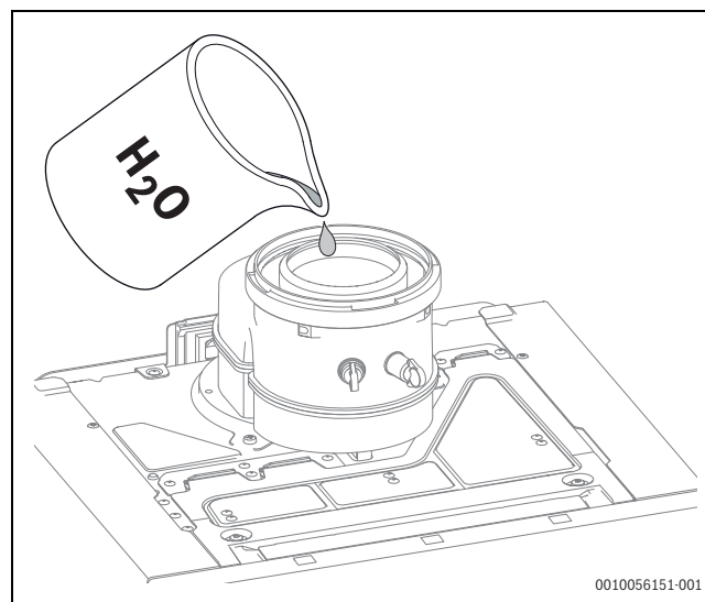
Bild 60 Kondensatsiphon mit Wasser füllen
