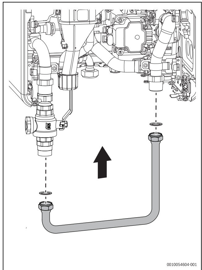
Bild 48 Bypassleitung installieren
