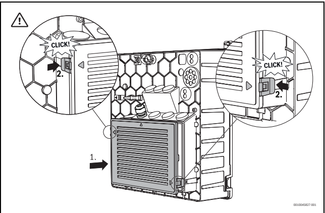
Bild 37 Korrekte Position der Abdeckung
