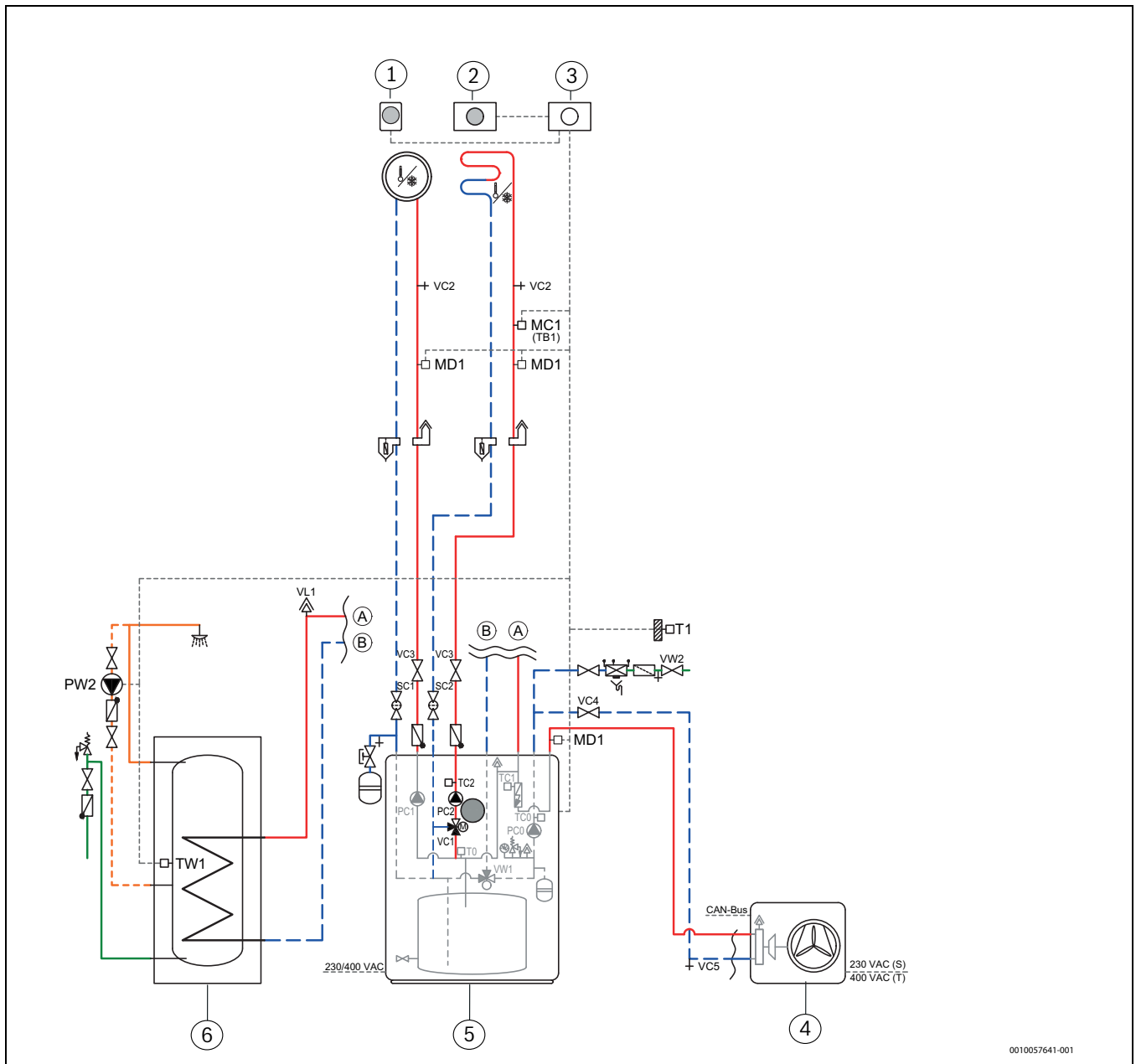
Bild 57 Anlagenlösung mit Zubehör Erweiterungs-Set 2HK intern
