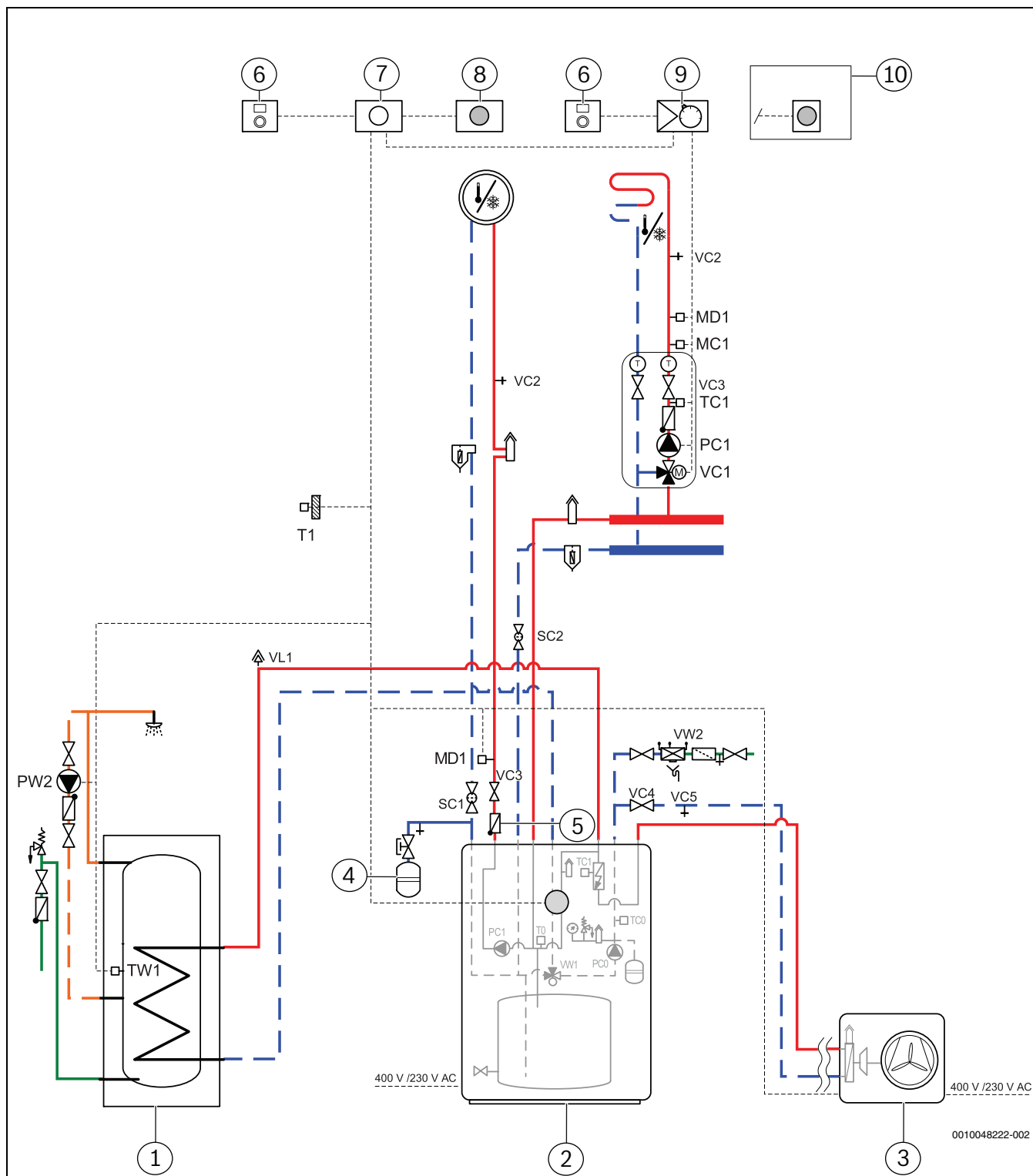
Bild 59 Anlage mit Außeneinheit, Inneneinheit mit integriertem Zuheizer und Pufferspeicher, einem ungemischten und einem gemischten Heizkreis
