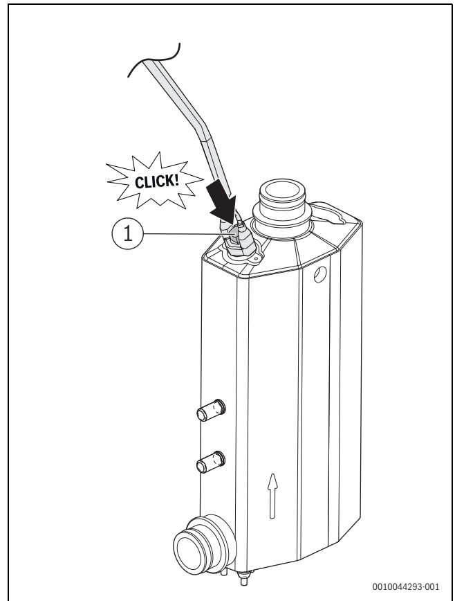
Bild 47 Elektrischer Zuheizer
