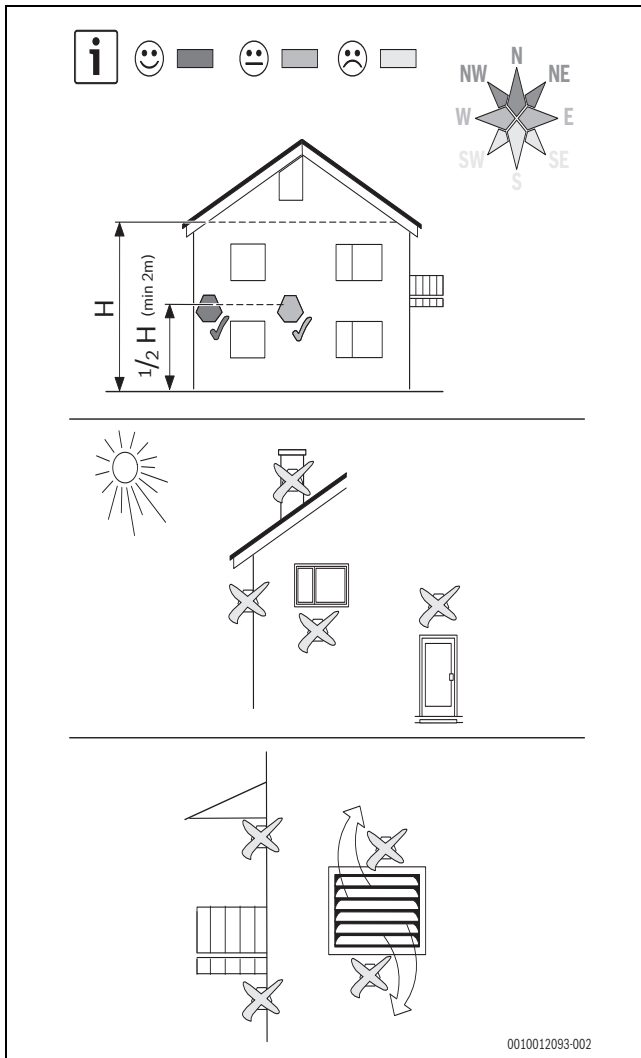
Bild 40 Position des Außentemperaturfühlers
