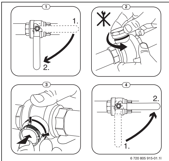
Bild 50 Filterventil reinigen
