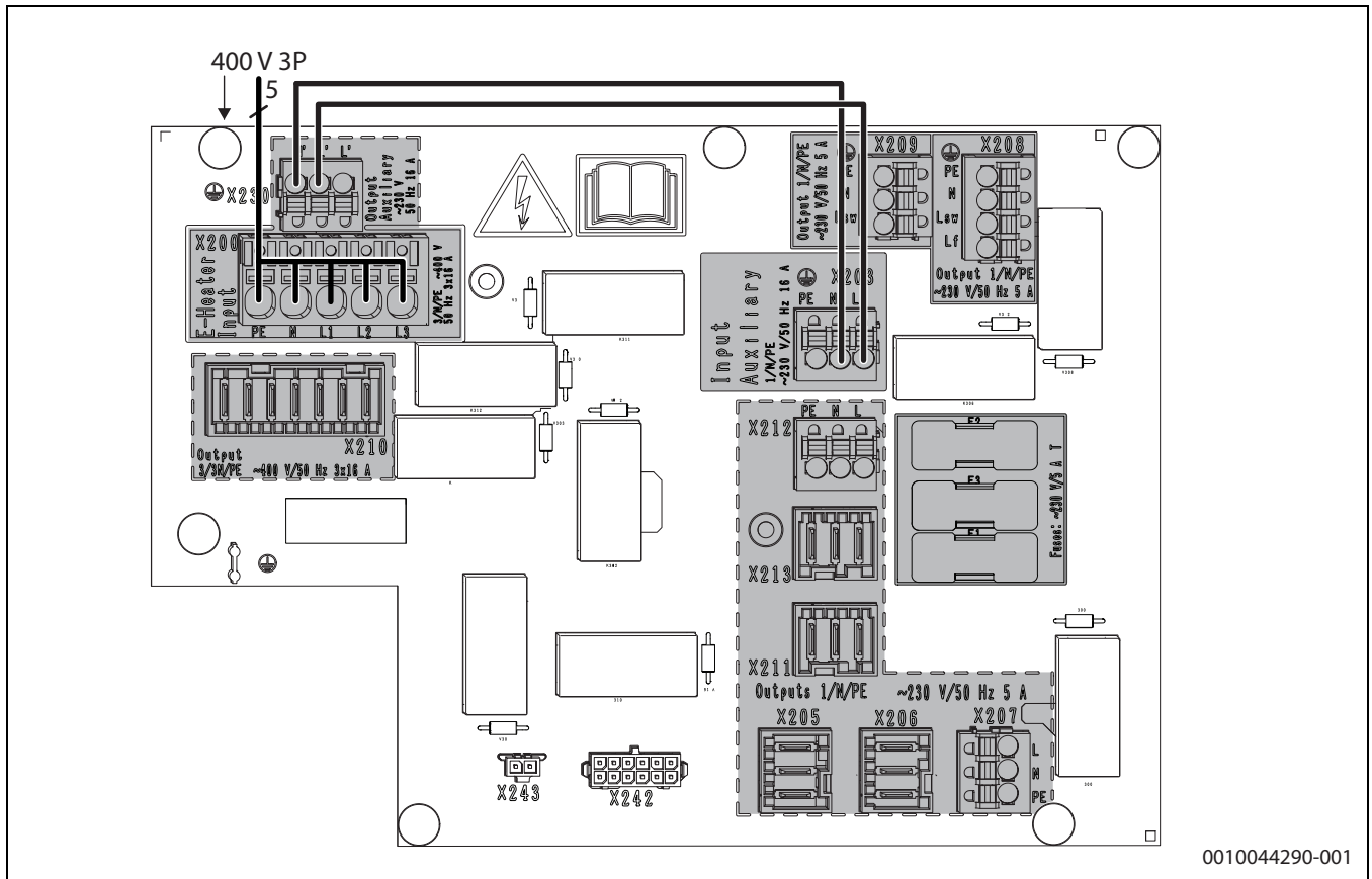
Bild 35 400 V Anschluss für den elektrischen Zuheizer mit gebrücktem 230 V Anschluss für Steuerung und Pumpen
