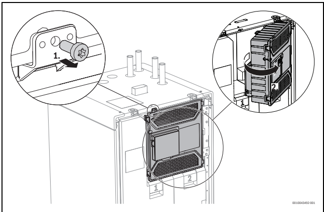
Bild 48 Elektronikbox
