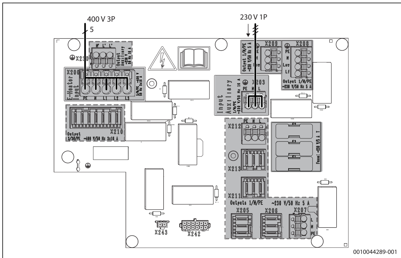
Bild 34 400 V Anschluss für den elektrischen Zuheizer, 230 V Anschluss für Steuerung und Pumpen
