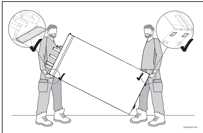
Bild 10 Inneneinheit anheben
