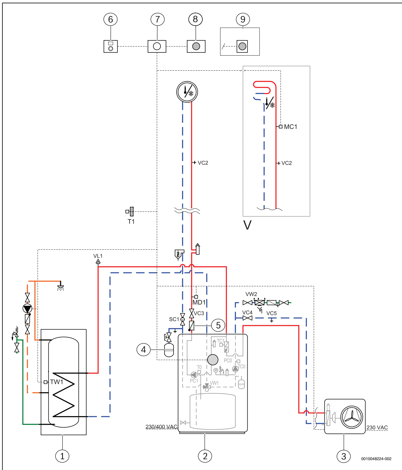
Bild 22 Anlagenlösung mit Außeneinheit, Inneneinheit mit integriertem Zuheiz- und Pufferspeicher und einem ungemischten Heizkreis
