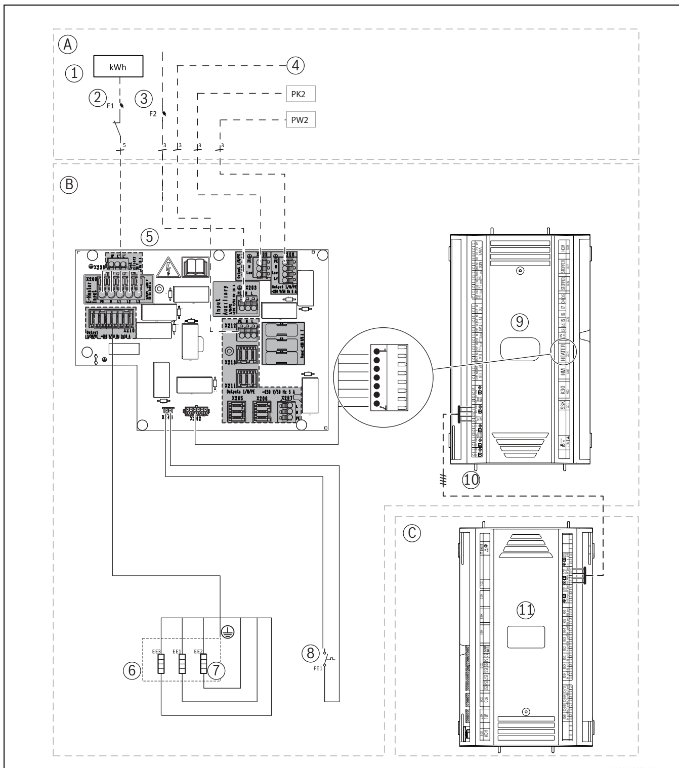
Bild 53 Spannungsversorgung Inneneinheit
