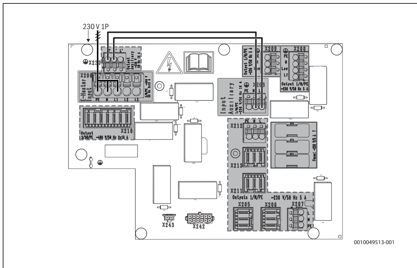
Bild 33 230 V Anschluss für den elektrischen Zuheizer mit gebrücktem 230 V Anschluss für Steuerung und Pumpen
