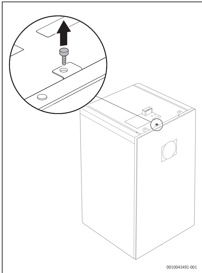
Bild 11 Sicherungsschraube lösen
