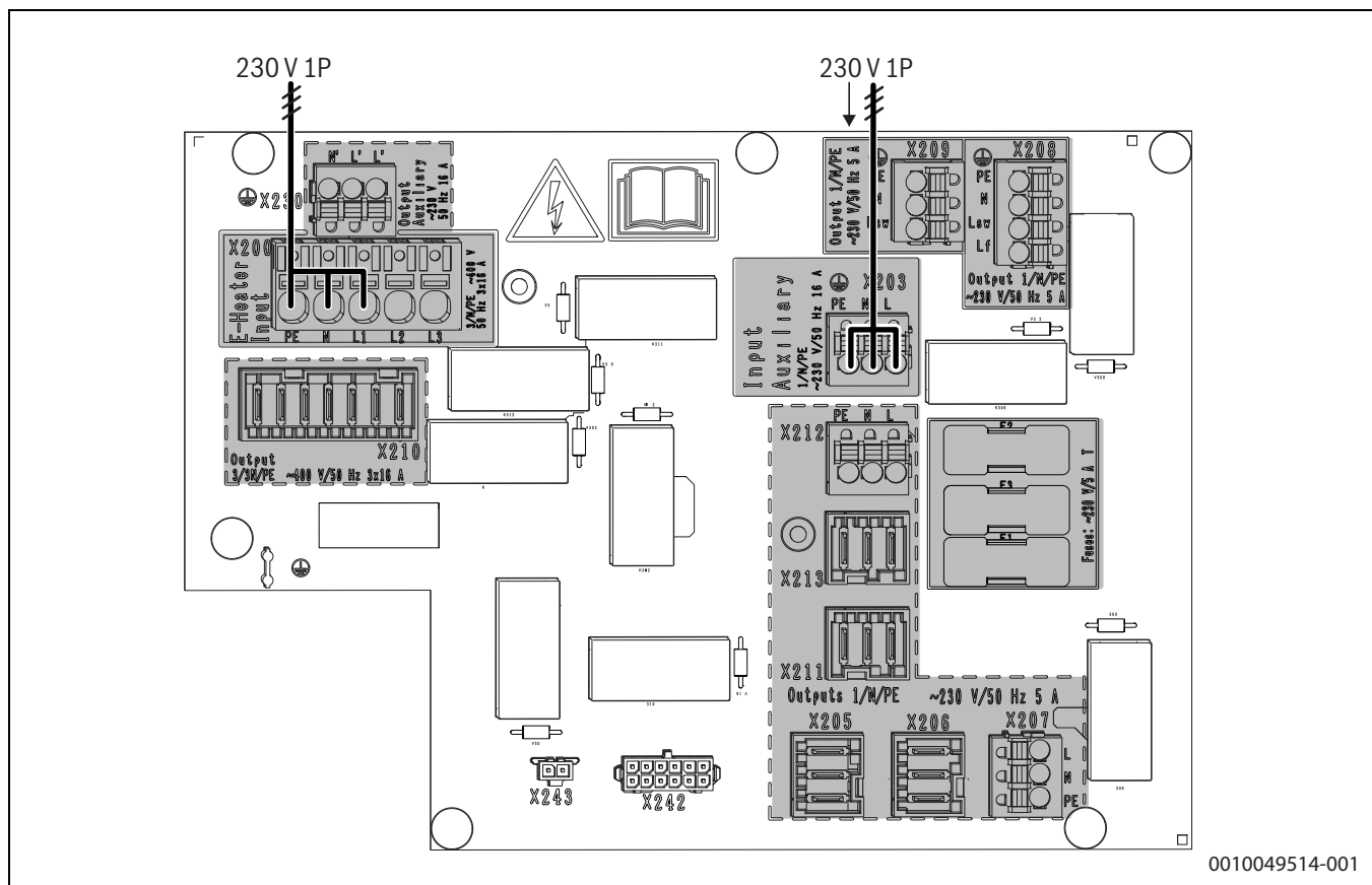
Bild 32 230 V Anschluss für den elektrischen Zuheizer, 230 V Anschluss für Steuerung und Pumpen
