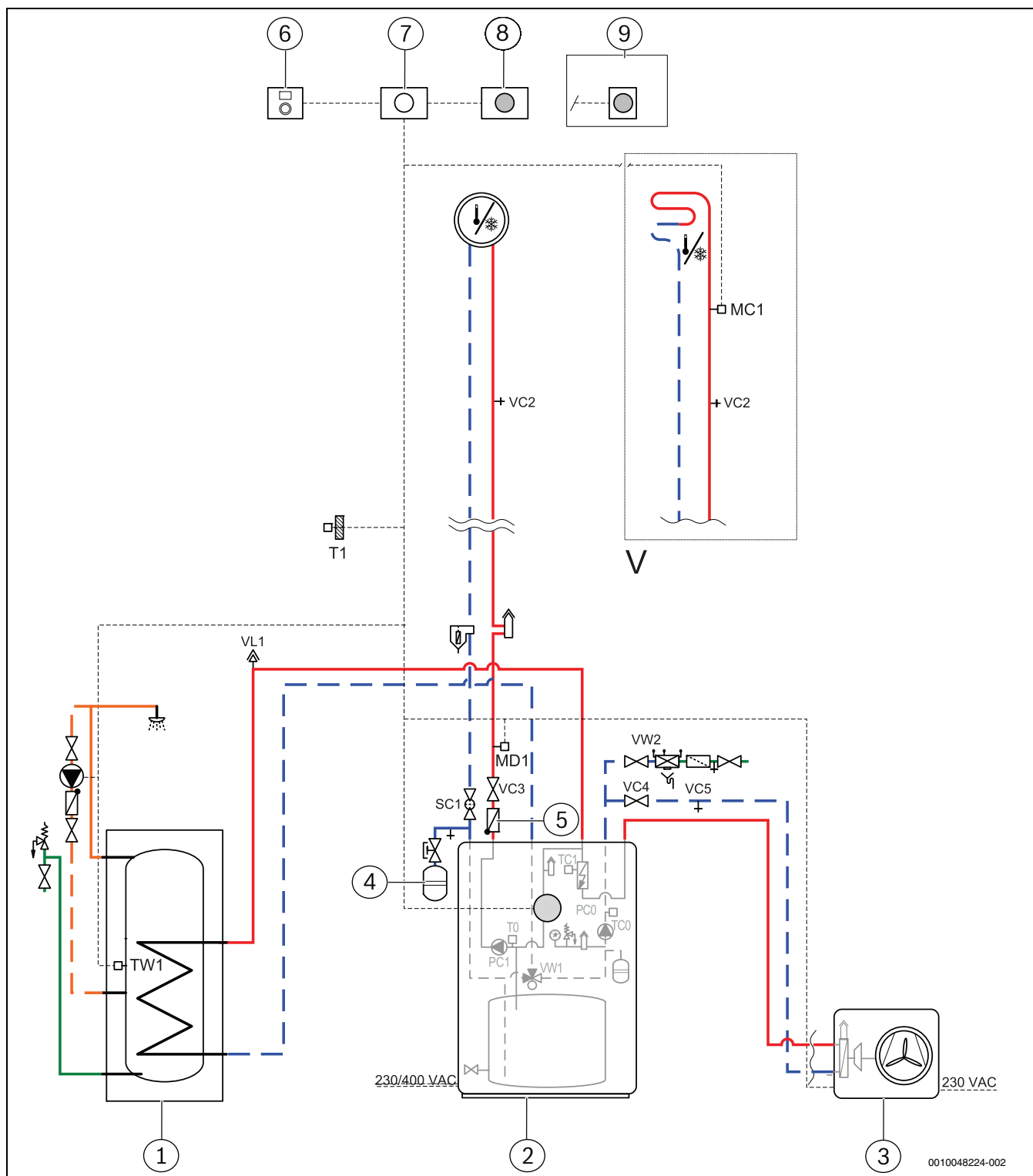
Bild 58 Anlage mit Außeneinheit, Inneneinheit mit integriertem Zuheizer, Pufferspeicher und einem ungemischten Heizkreis
