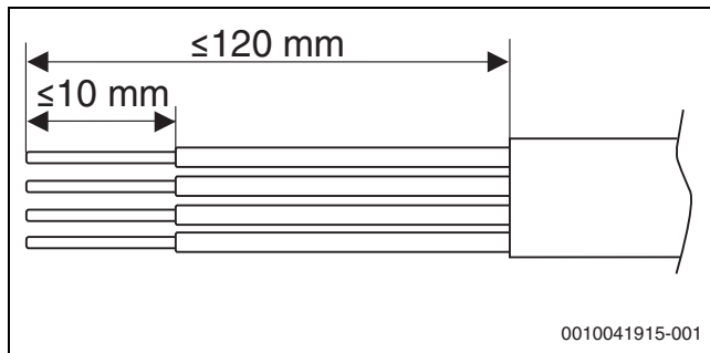
Bild 38 Abisolierung CAN-BUS
