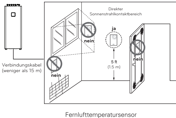
Fernlufttemperatursensor
