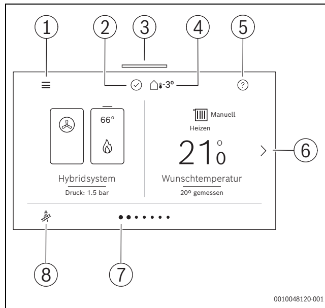
Bild 3 Bedienfeld
