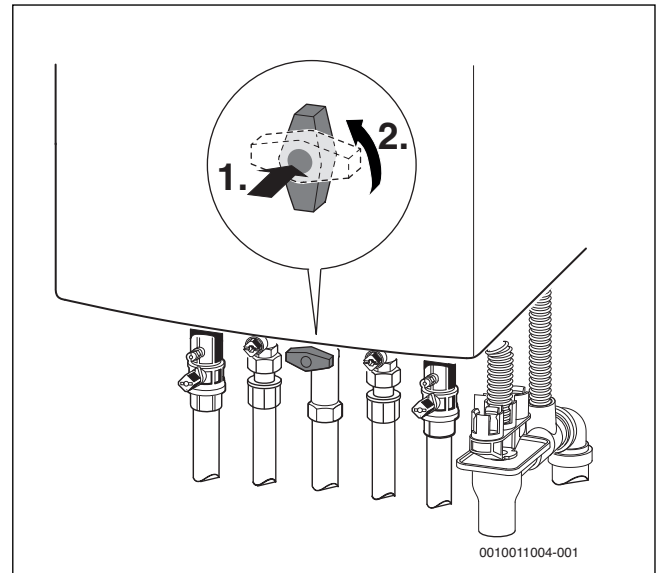
Bild 2 Gashahn öffnen
