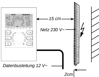
Bild 1: Mindestabstände bei der Elektroinstallation
