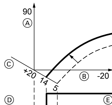
Abb. 54 Beispiel 2: Änderung des reduzierten Raumtemperatur-Sollwerts von 5 °C auf 14 °C
