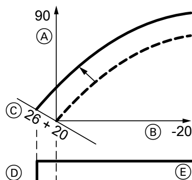
Abb. 53 Beispiel 1: Änderung des Raumtemperatur-Sollwerts von 20 auf 26 °C
