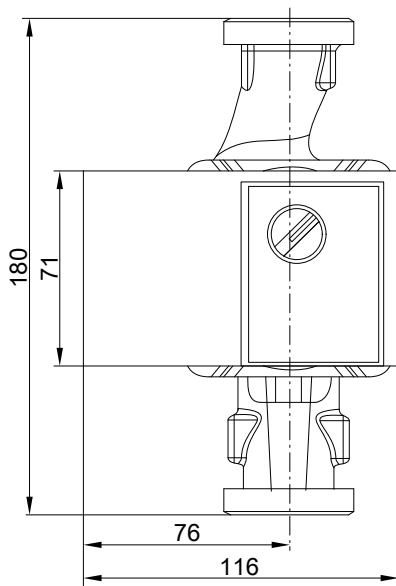
Abmessungen Stratos 40/1-4
