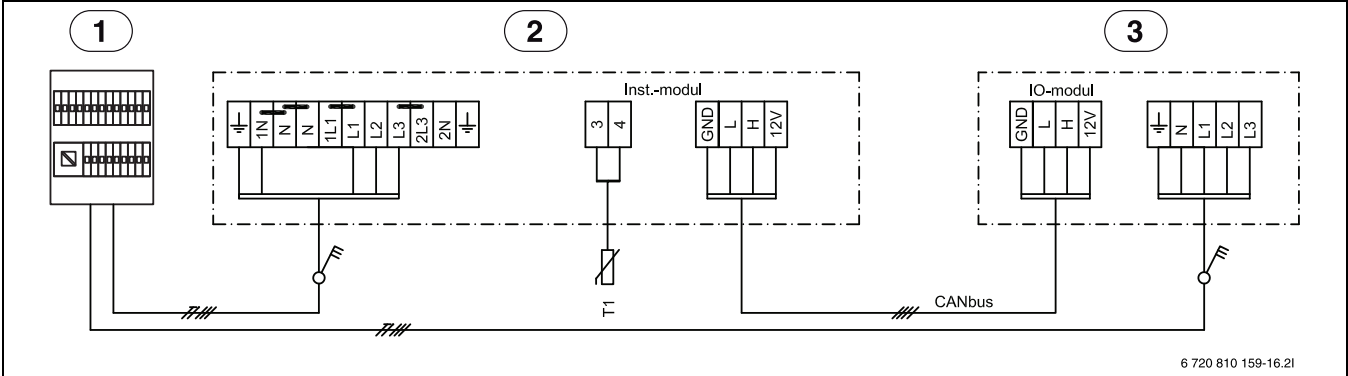
Bild 51 Schaltplan 3 N~
