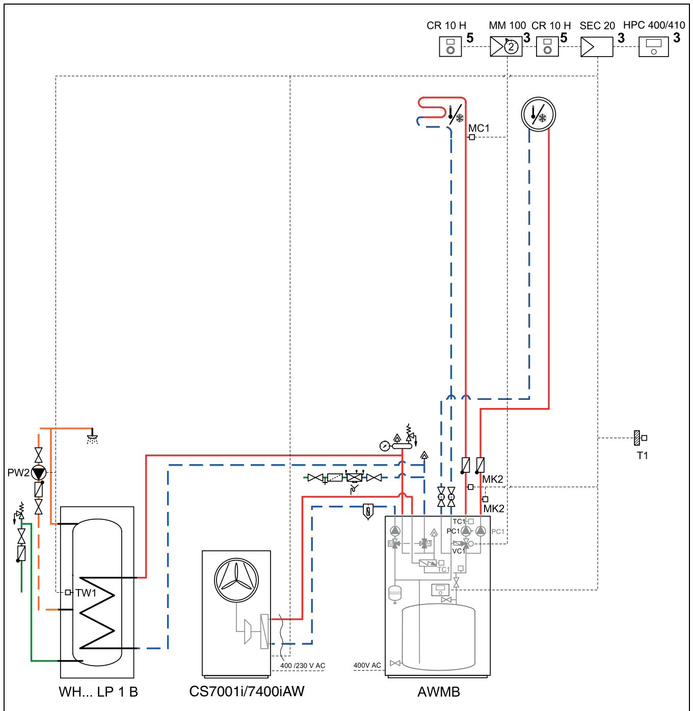
Bild 48 Wärmepumpe, Inneneinheit mit einem gemischten und einem ungemischten Kreis
