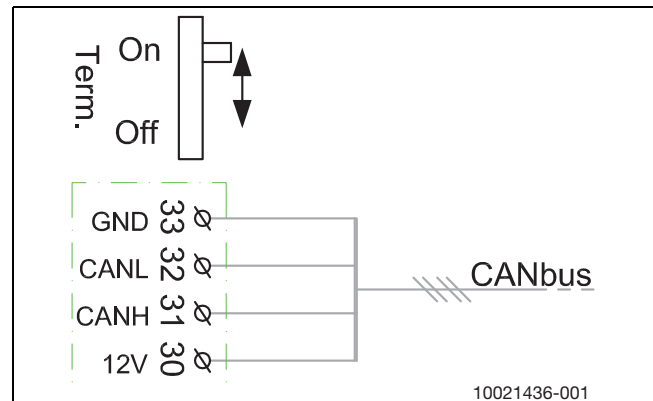
Bild 15 CAN-BUS-Terminierung
