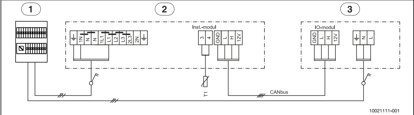
Bild 52 Schaltplan 1N~ 1)
